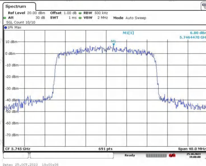
11AX20ISO_Ant2_5745
