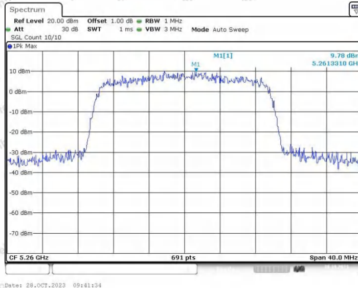
11AX20SISO_Ant2_5260
