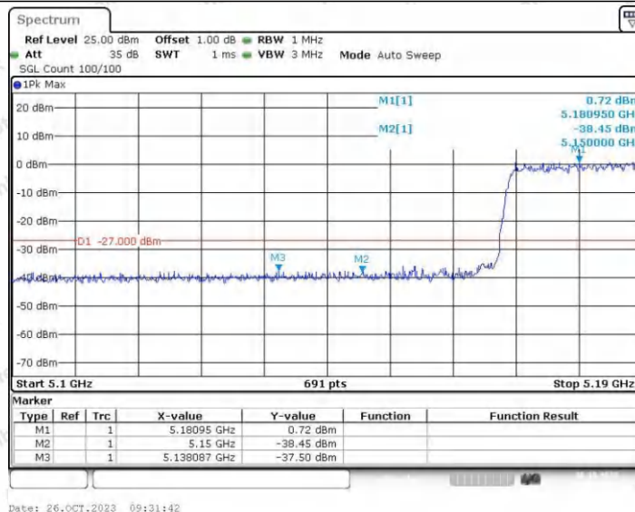
11AX80SISO_Ant1_Low_5210
