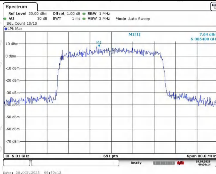
11AX40ISO_Ant1_5310
