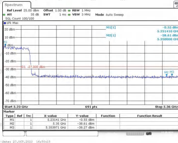
11AX80SISO_Ant1_Low_5290
