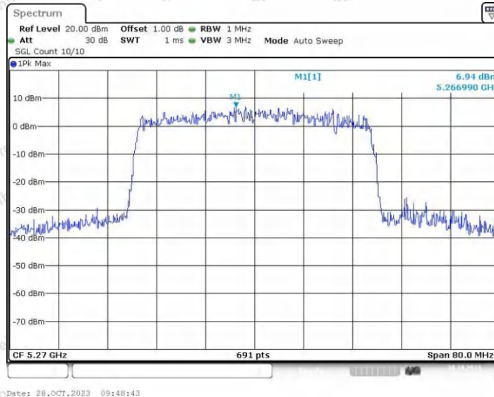
11AX40ISO_Ant2_5270
