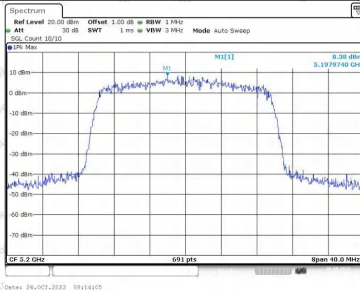
11AX20SISO_Ant2_5200
