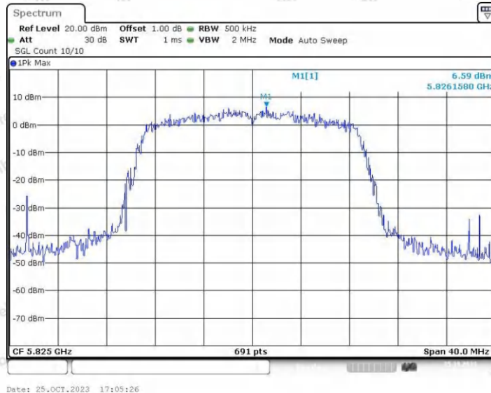
11N20SISO_Ant2_5825
