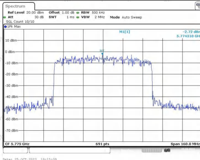
11AX80ISO_Ant2_5775
