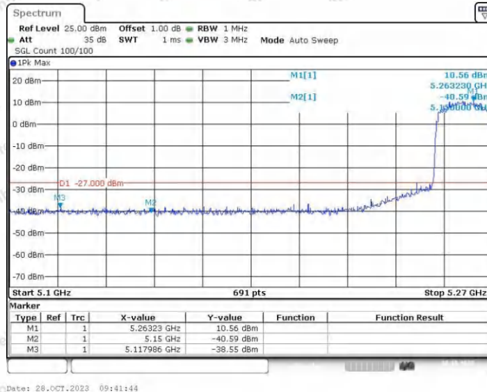
11AX20SISO_Ant2_Low_5260
