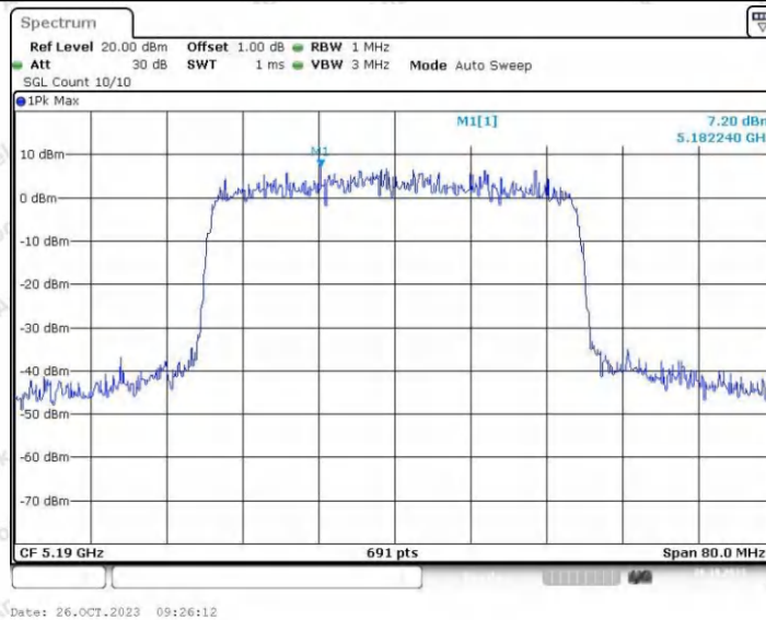
11AX40ISO_Ant2_5190
