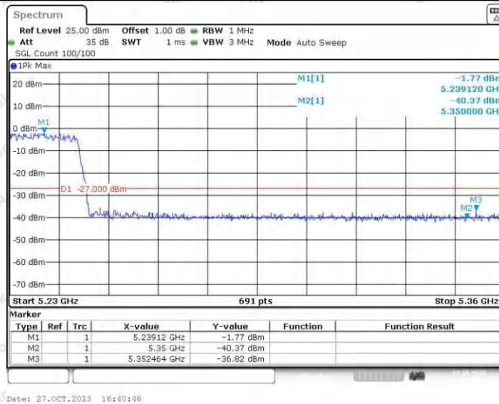
11AC80SISO_Ant1_Low_5290
