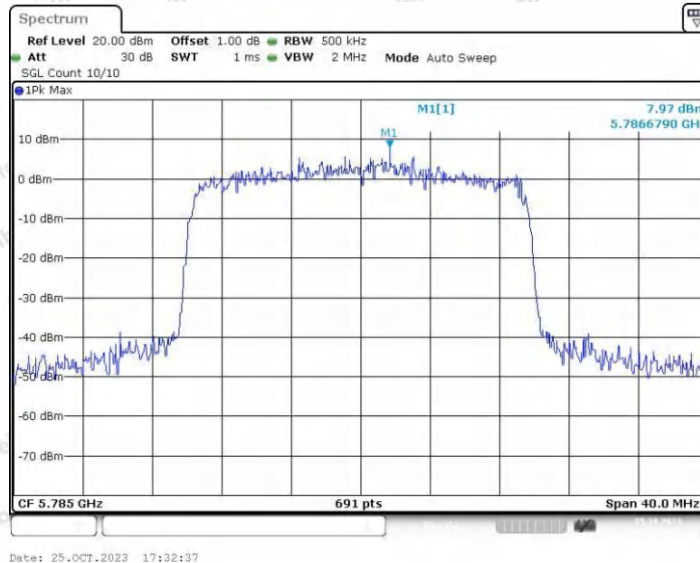
11AX20SISO_Ant2_5785
