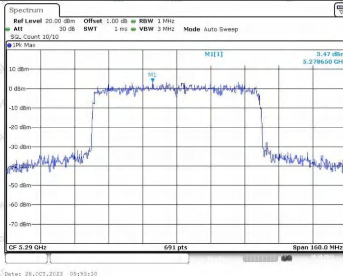
11AX80ISO_Ant2_5290
