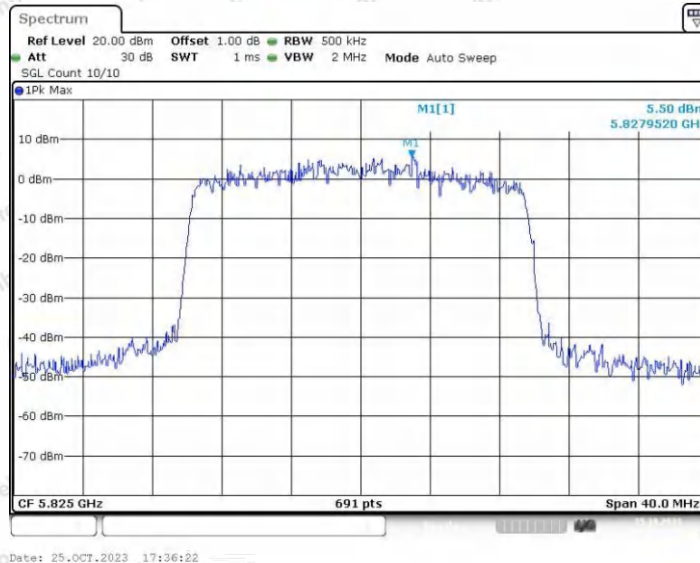
11AX20ISO_Ant2_5825
