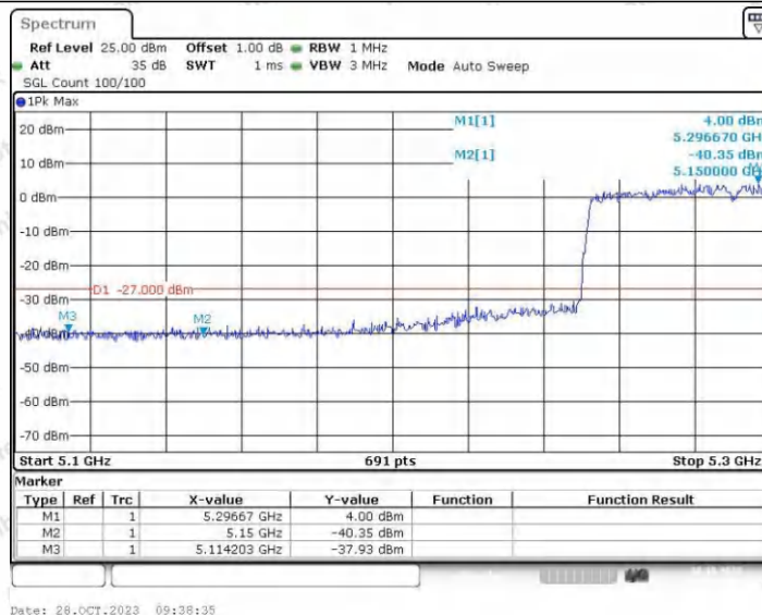
11AC80SISO_Ant1_Low_5290
