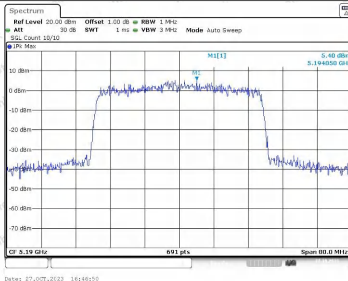
11AX40ISO_Ant2_5190
