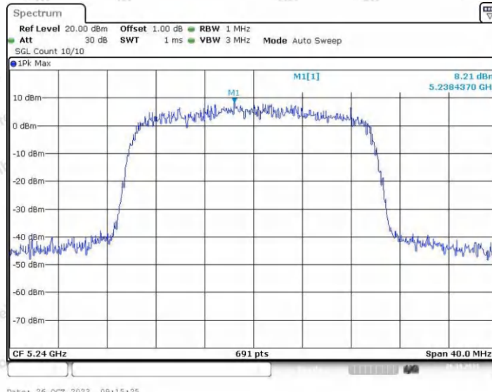
11AX20SISO_Ant2_5240
