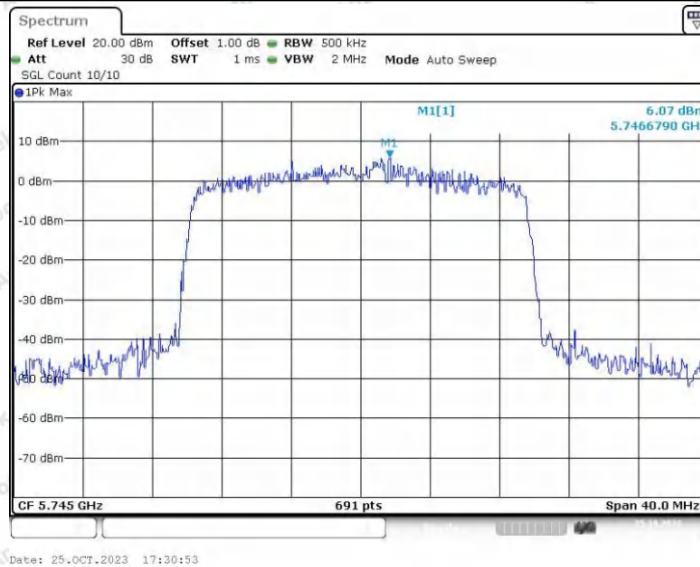
11AX20ISO_Ant2_5745
