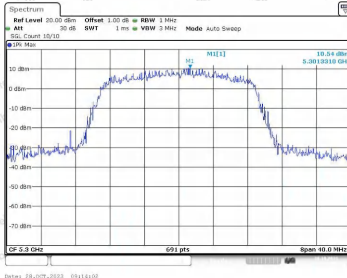
11N20SISO_Ant2_5300
