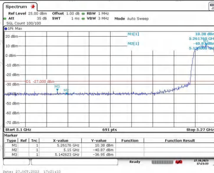
11A_Ant1_Low_5260
