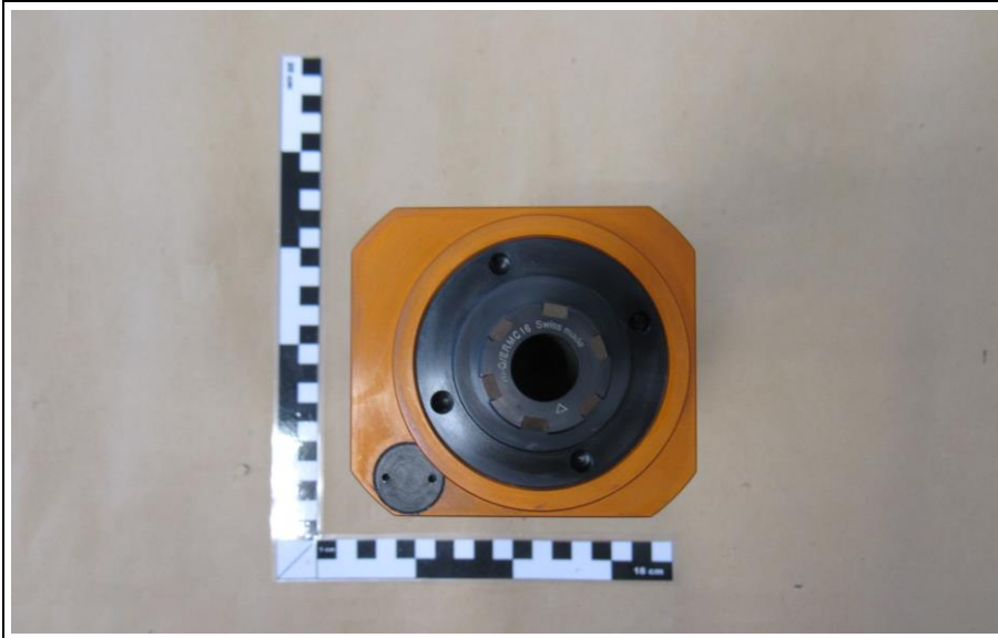
EUT FRONT
