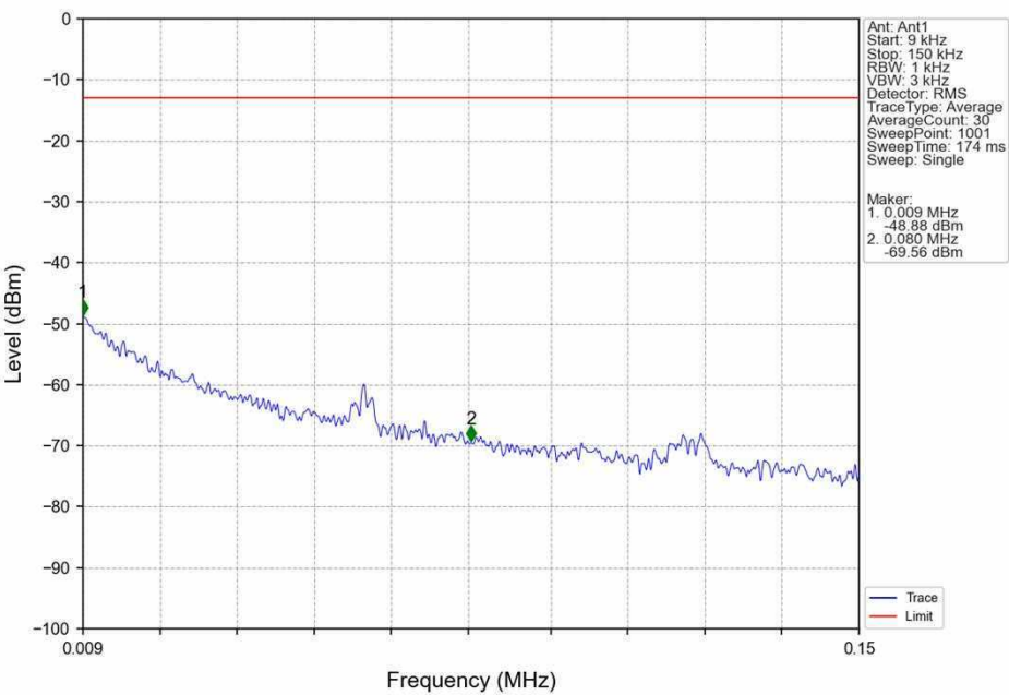
Band12 5MHz 16QAM MCH 707.5MHz RB 1 0 NTNV
