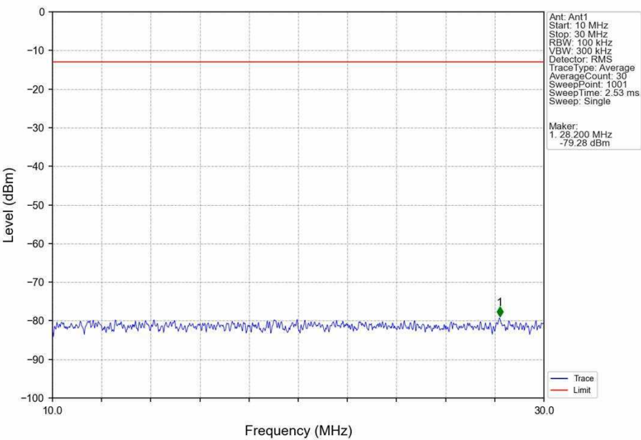
Band12 5MHz QPSK LCH 701.5MHz RB 1 0 NTN
