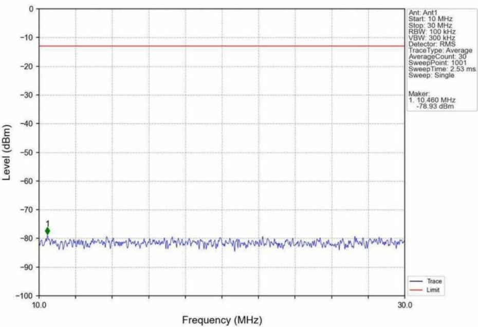
Band12 10MHz 16QAM MCH 707.5MHz RB 1 0 NTV
