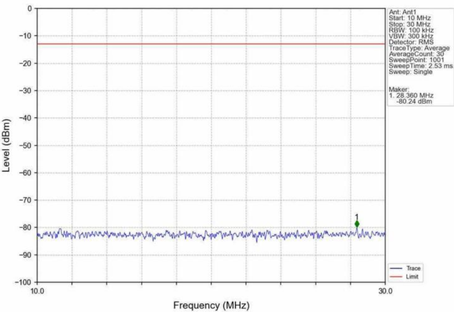
Band4 10MHz QPSK HCH 1750MHz RB 1 0 NTN
