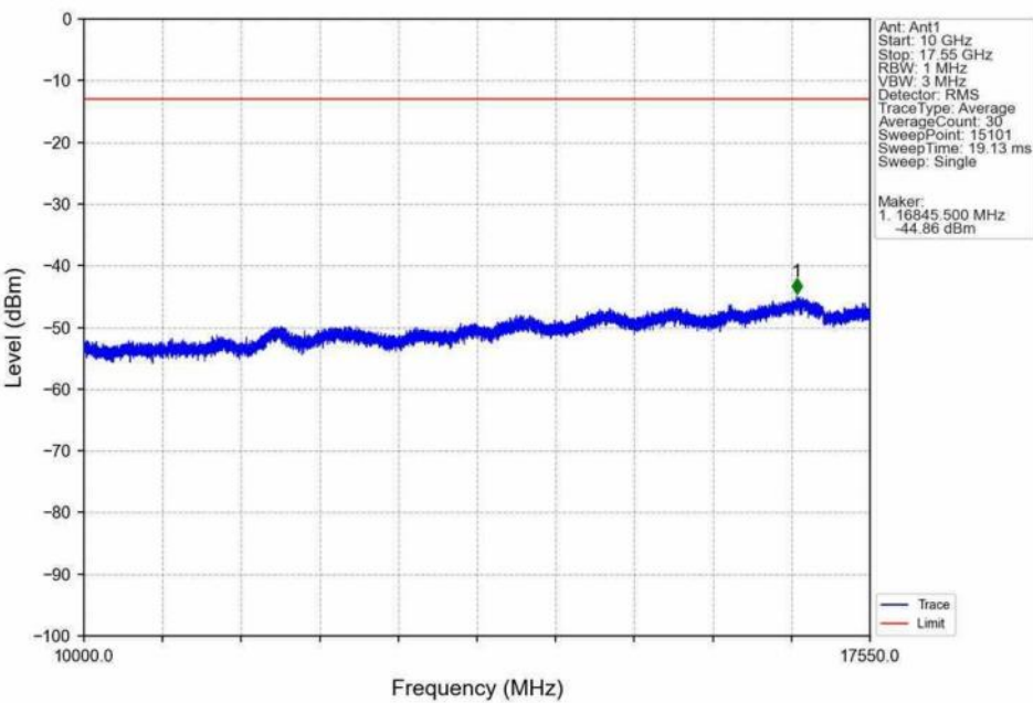
Band4 10MHz 16QAM HCH 1750MHz RB 1 49 NTNV
