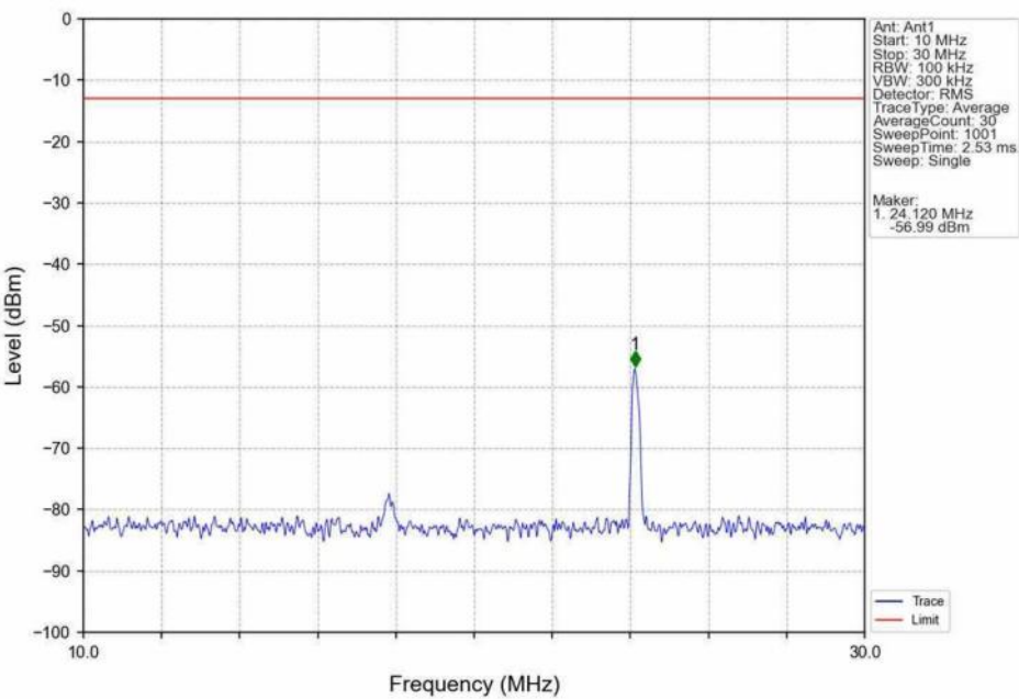
Band4 20MHz QPSK MCH 1732.5MHz RB 1 0 NTNV
