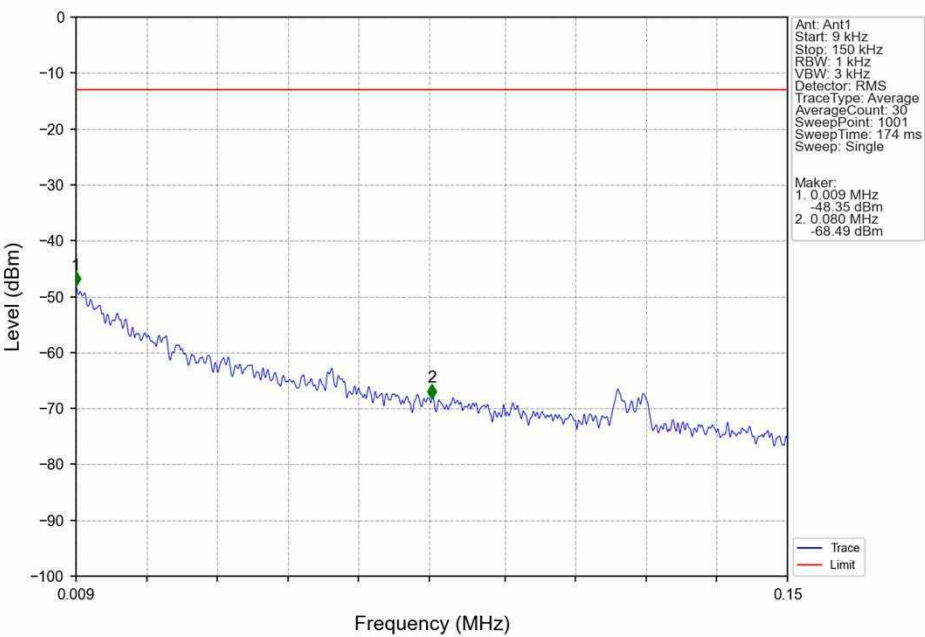
Band4 15MHz 16QAM LCH 1717.5MHz RB 1 0 NTV
