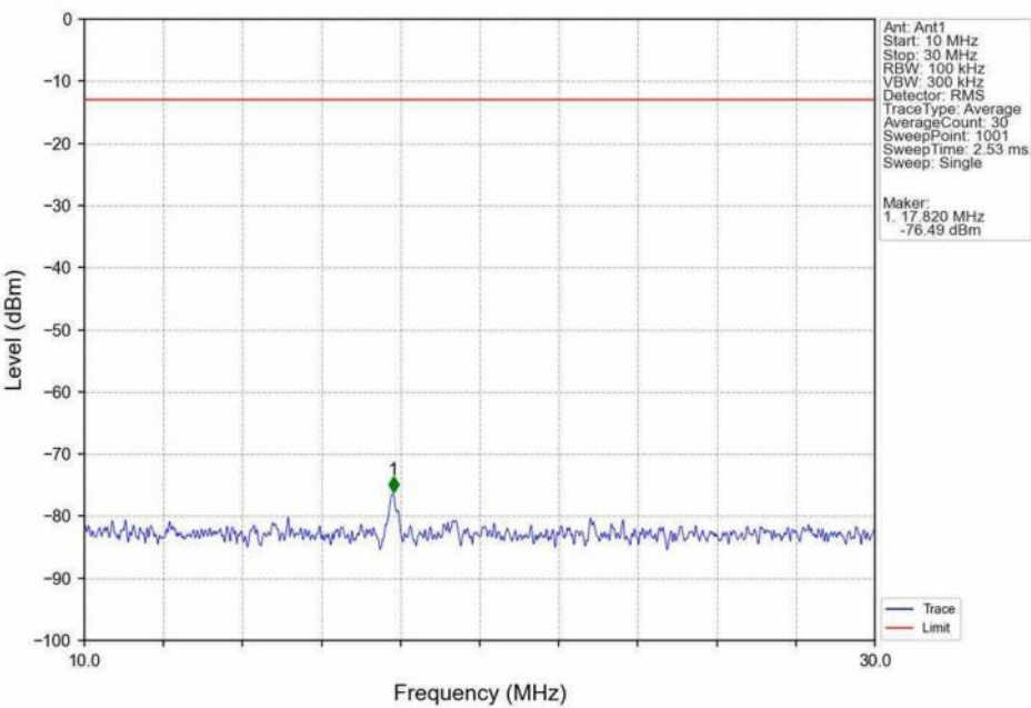
Band4 20MHz QPSK HCH 1745MHz RB 1 0 NTN
