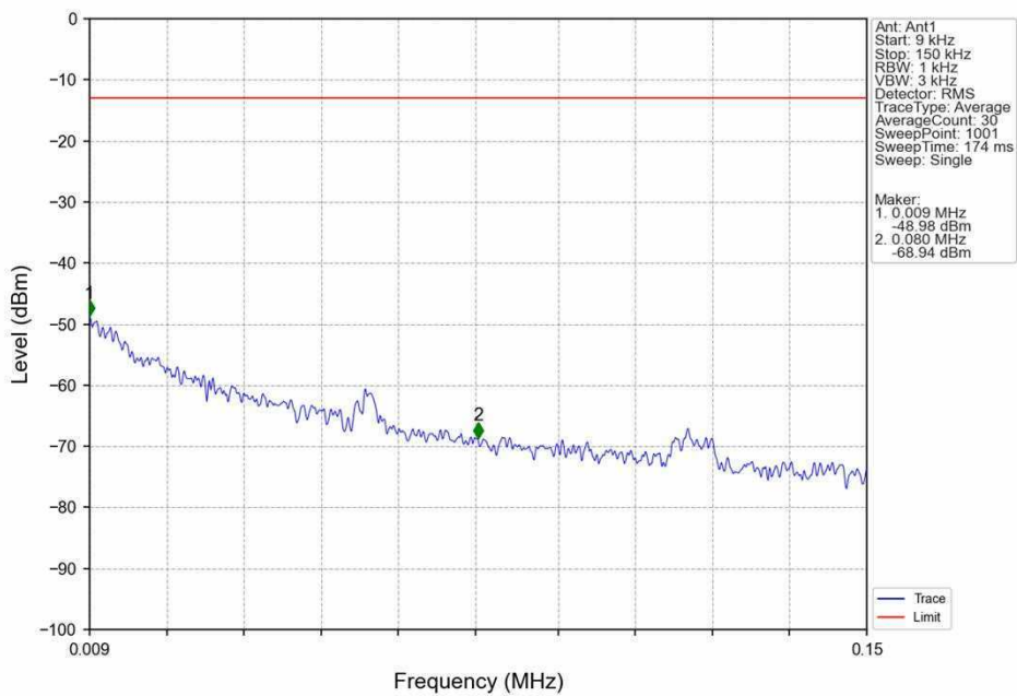
Band4 20MHz 16QAM LCH 1720MHz RB 1 0 NTN
