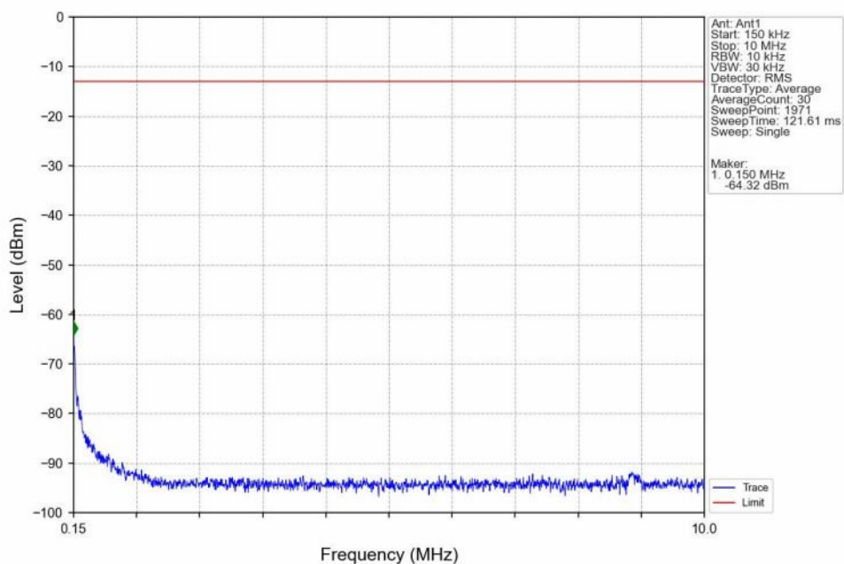
Band2_20MHz_16QAM_LCH_1860MHz_RB_1_0_NTNV
