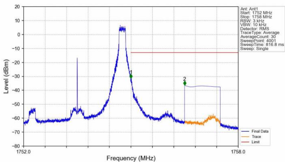
Band4_3MHz_QPSK_HCH_1753.5MHz_RB_1_14_NTNV
