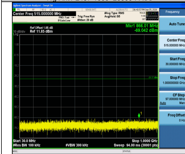
11g-Ant1-2462-30~1000-PASS
