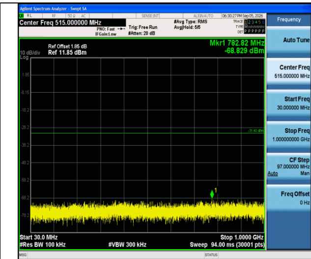
11g-Ant1-2437-30~1000-PASS
