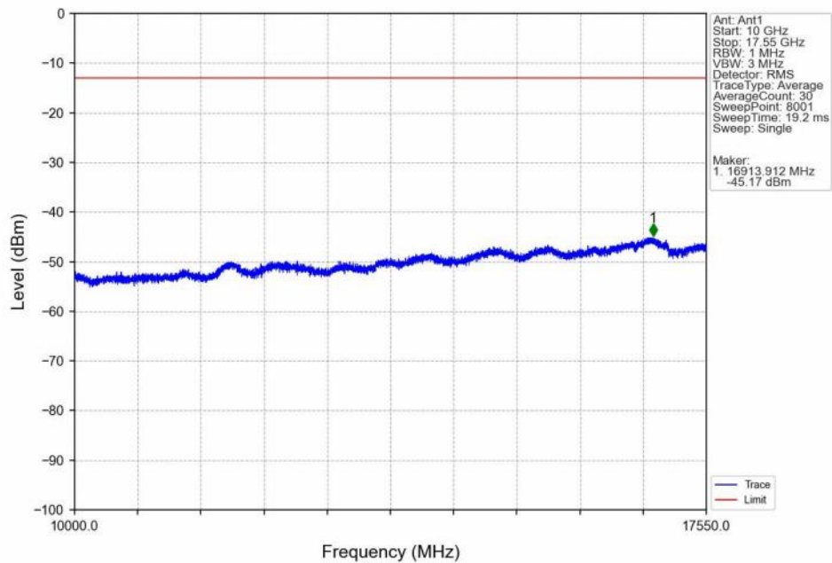
Band4_10MHz_QPSK_HCH_1750MHz_RB_1_49_NTNV
