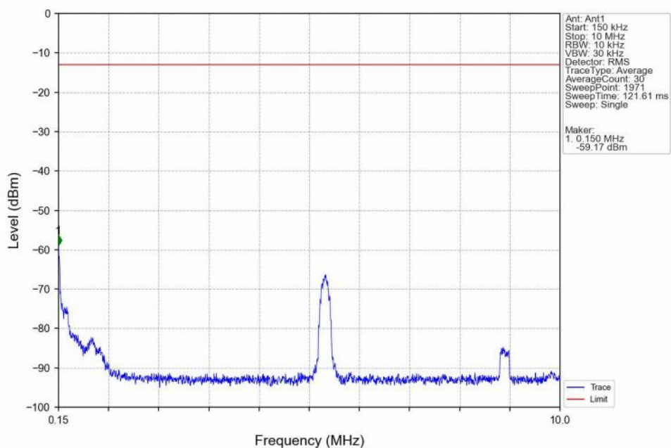
Band4_20MHz_16QAM_LCH_1720MHz_RB_1_0_NTNV
