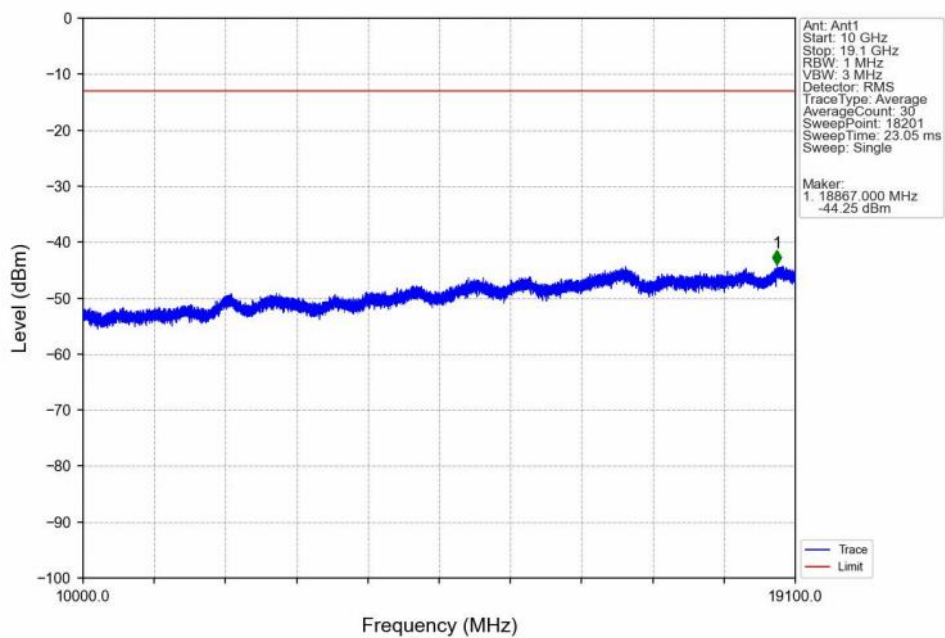
Band2_3MHz_QPSK_HCH_1908.5MHz_RB_1_14_NTNV
