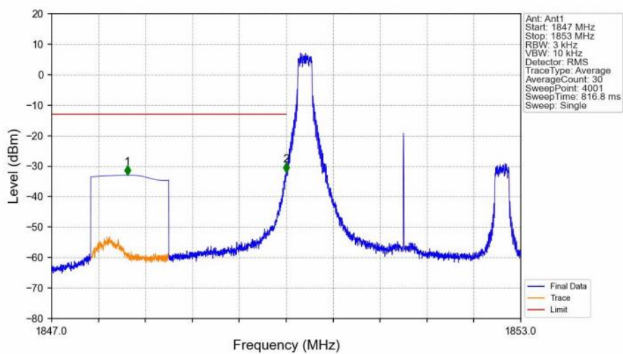
Band2_3MHz_QPSK_LCH_1851.5MHz_RB_1_0_NTNV
