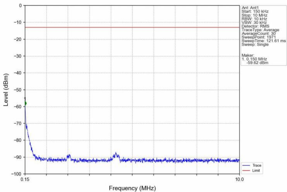
Band2_5MHz_QPSK_MCH_1880MHz_RB_1_0_NTNV
