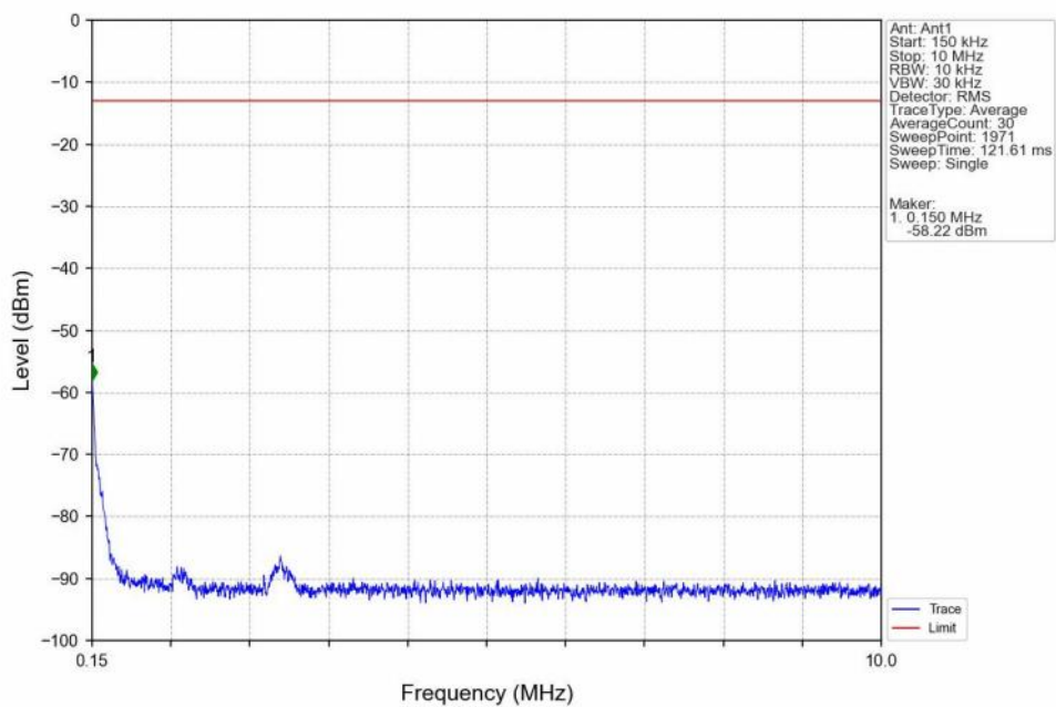
Band2_3MHz_QPSK_MCH_1880MHz_RB_1_0_NTNV
