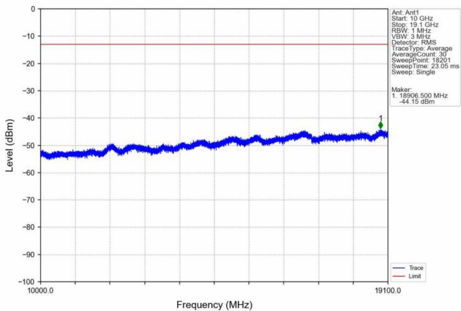
Band2_10MHz_16QAM_HCH_1905MHz_RB_1_49_NTNV
