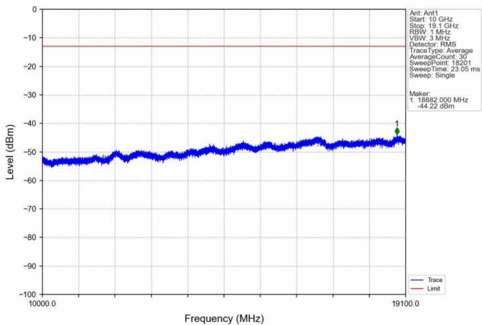
Band2_10MHz_QPSK_HCH_1905MHz_RB_1_49_NTNV
