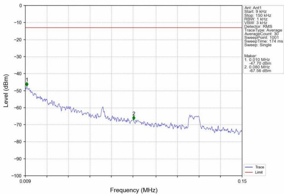
Band2_10MHz_16QAM_LCH_1855MHz_RB_1_0_NTNV
