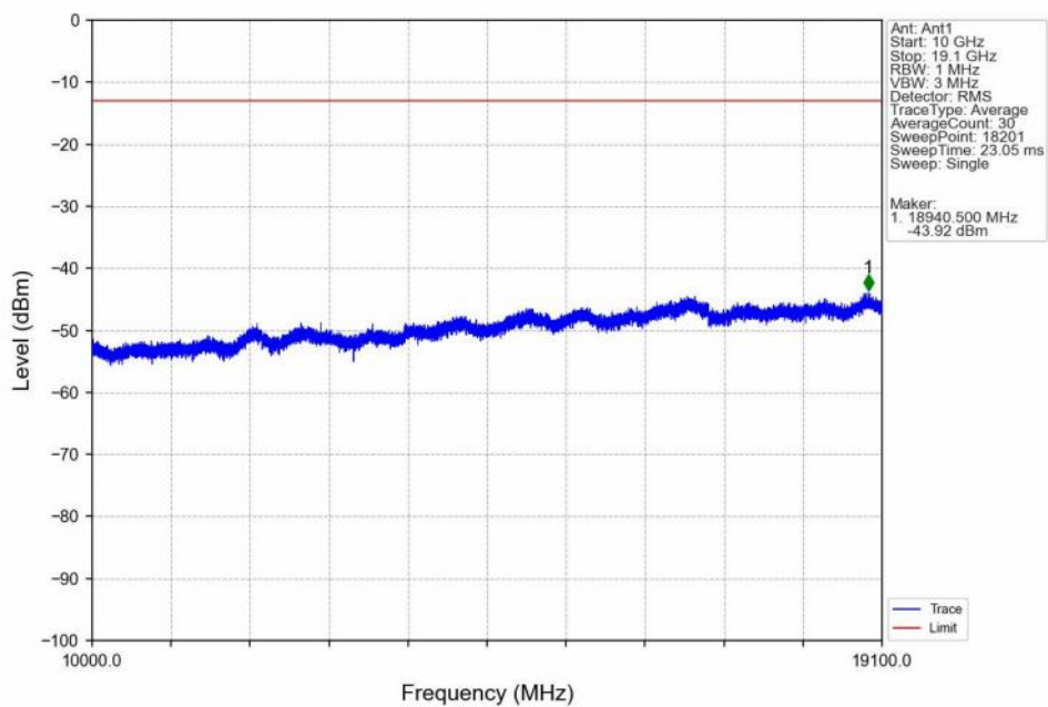
Band2_20MHz_16QAM_HCH_1900MHz_RB_1_99_NTNV
