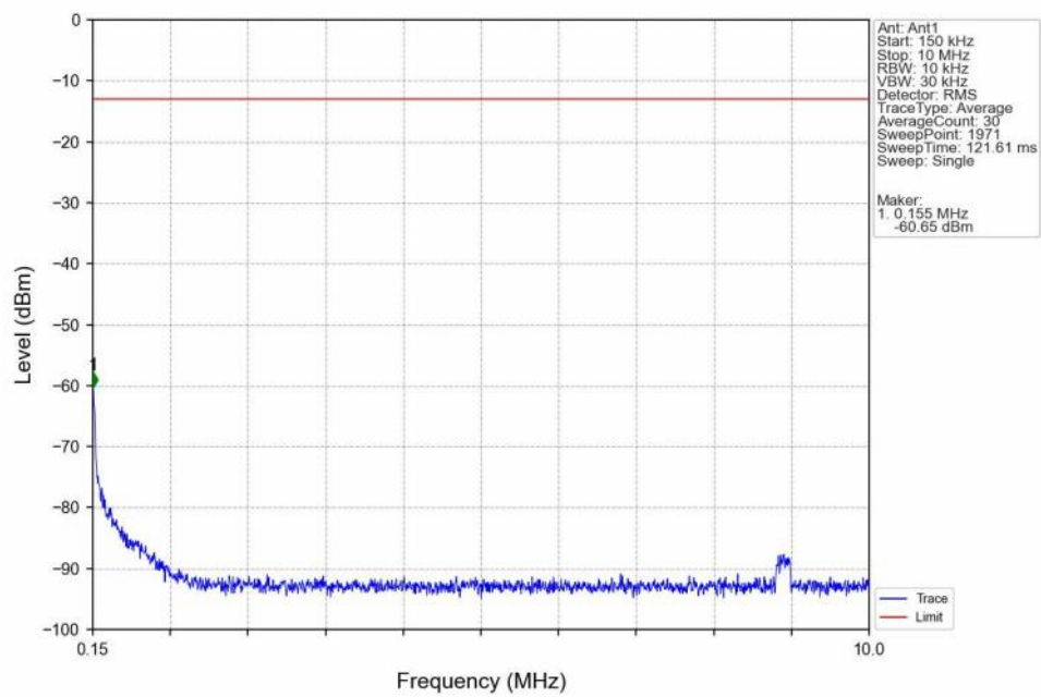
Band2_20MHz_16QAM_LCH_1860MHz_RB_1_0_NTNV
