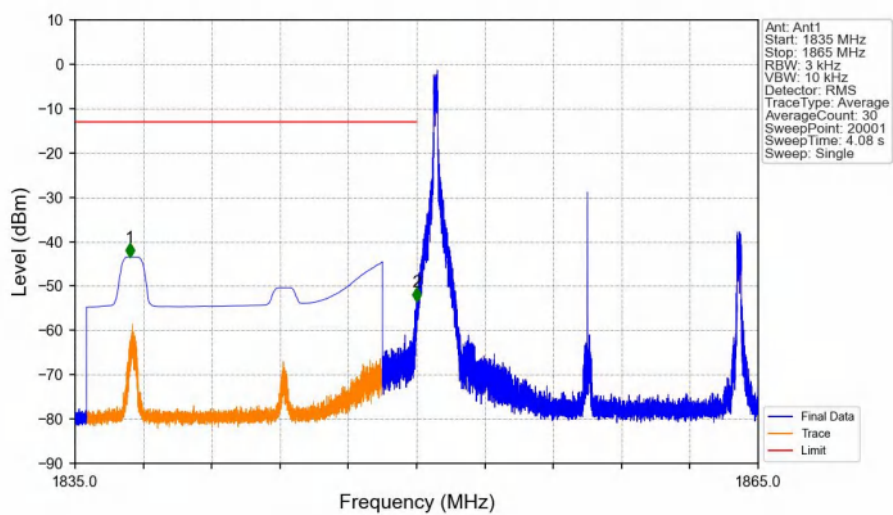
Band2_15MHz_QPSK_LCH_1857.5MHz_RB_1_0_NTNV
