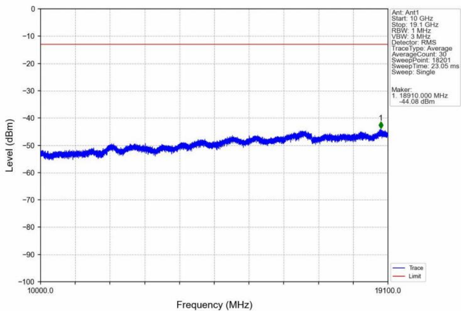
Band2_15MHz_QPSK_HCH_1902.5MHz_RB_1_74_NTNV
