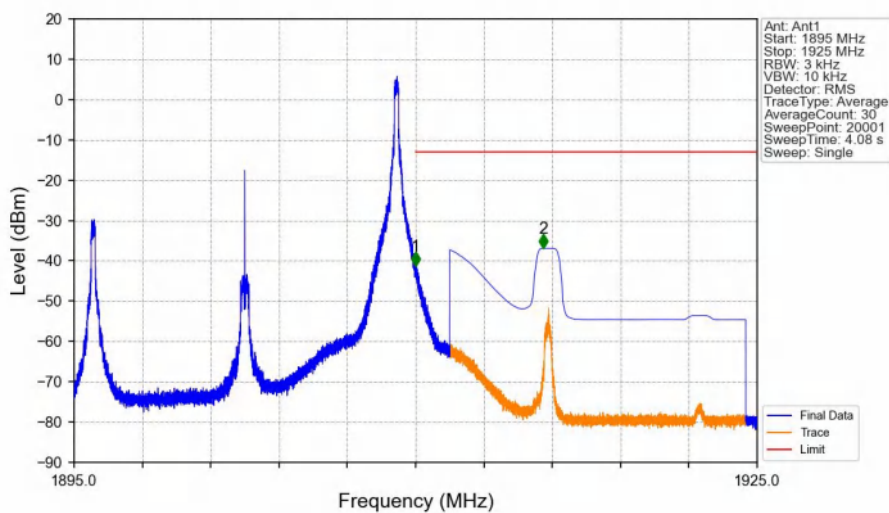
Band2_15MHz_QPSK_HCH_1902.5MHz_RB_1_74_NTNV
