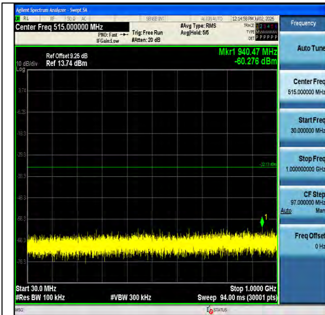
11g-Ant1-2462-30~1000-PASS
