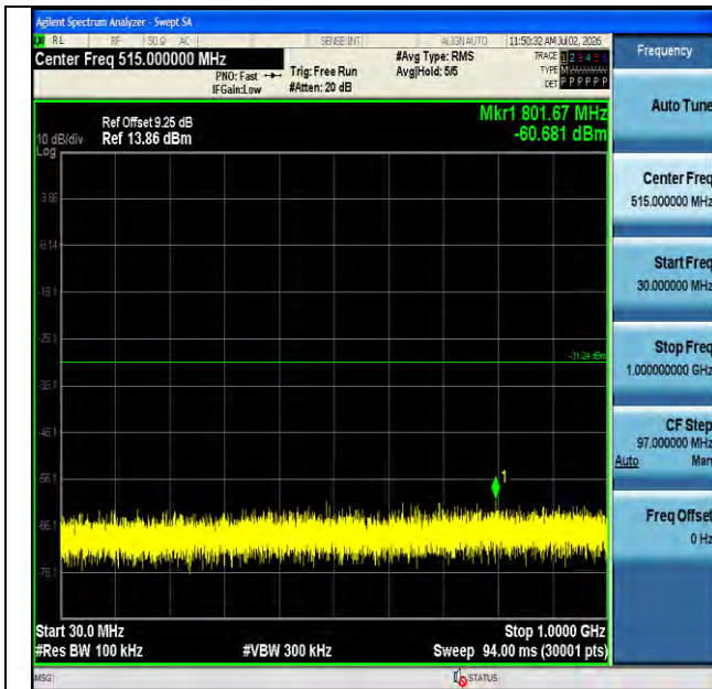
11g-Ant1-2412-30~1000-PASS
