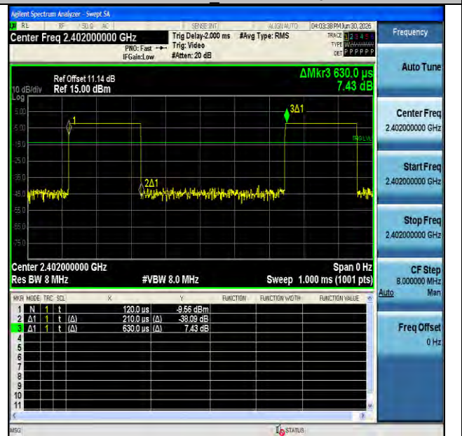
NTNV-BLE_2M-Ant1-2402
