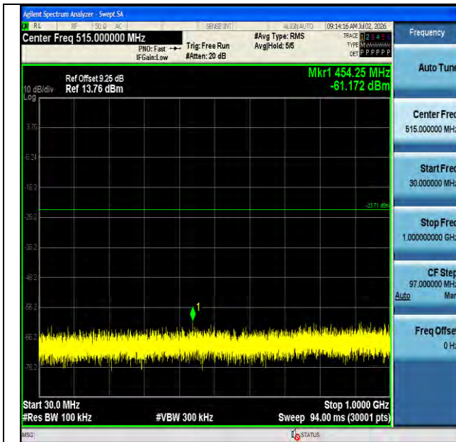
BLE_2M-Ant1-2480-30~1000-PASS
