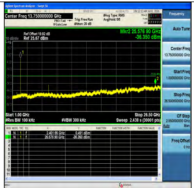
BLE 2M-Ant1-2402-1000~26500-PASS
