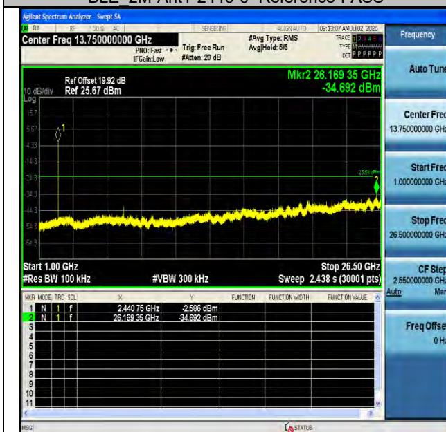
BLE 2M-Ant1-2440-1000~26500-PASS
