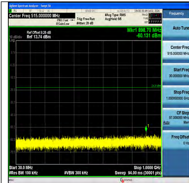
BLE 1M-Ant1-2440-30~1000-PASS
