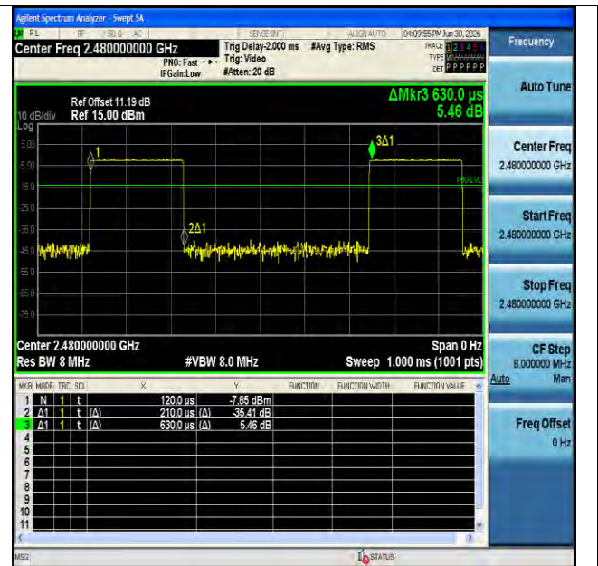
NTNV-BLE_2M-Ant1-2480
