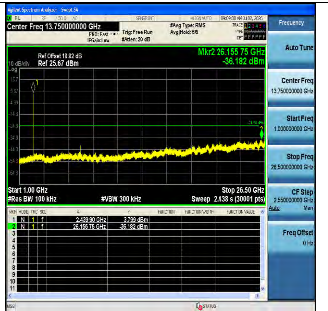
BLE 1M-Ant1-2440-1000~26500-PASS
