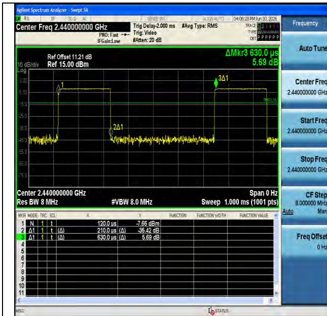
NTNV-BLE_2M-Ant1-2440
