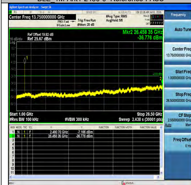
BLE 1M-Ant1-2480-1000~26500-PASS
