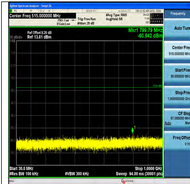
BLE 2M-Ant1-2402-30~1000-PASS
