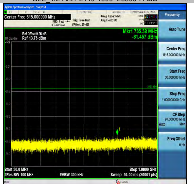
BLE 1M-Ant1-2480-30~1000-PASS
