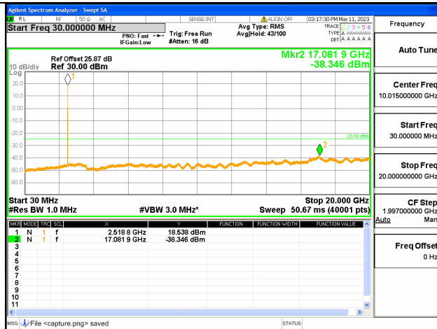
Band7C-30M-20G / 20+10MHz / 1RB+1RB / QPSK / Low CH
