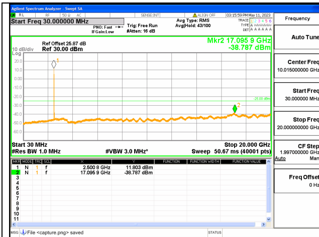
Band7C-30M-20G / 20+10MHz / 1RB+1RB / QPSK / Low CH
