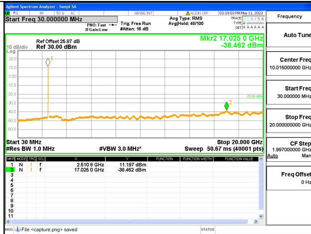
Band7C-30M-20G / 20+10MHz / 100RB+50RB / QPSK / Low CH
