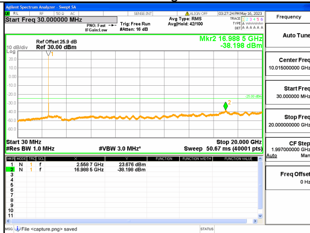
Band7C-30M-20G / 20+10MHz / 1RB+1RB/ QPSK / High CH
