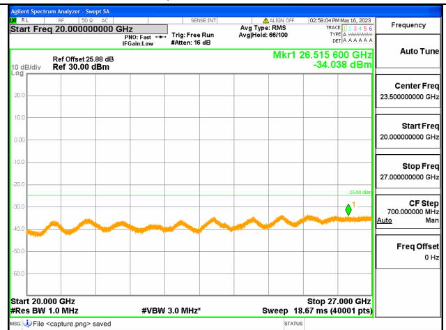
Band7C-20G-27G / 20+10MHz / 100RB+50RB/ QPSK / Mid CH
