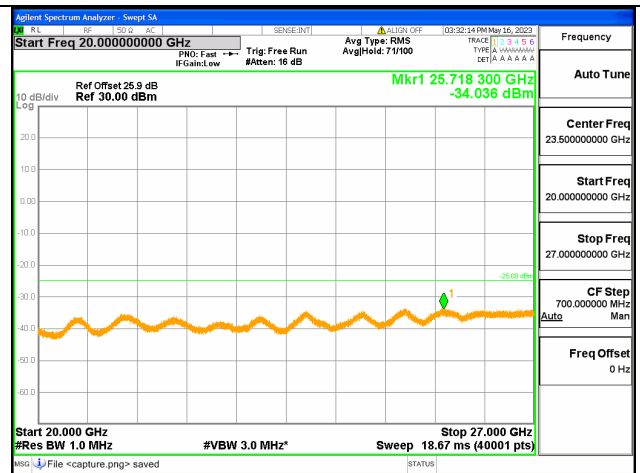
Band7C-20G-27G / 15+20MHz / 1RB+1RB/ QPSK / High CH
