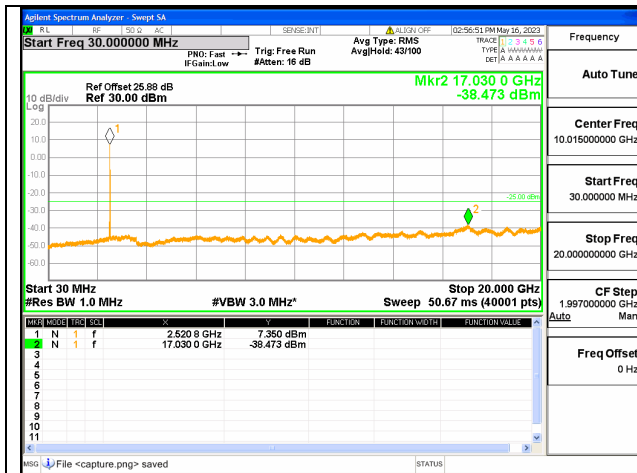
Band7C-30M-20G / 20+10MHz / 1RB+1RB/ QPSK / Mid CH
