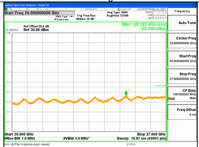
Band7C-20G-27G / 15+10MHz / 75RB+50RB/ QPSK / High CH
