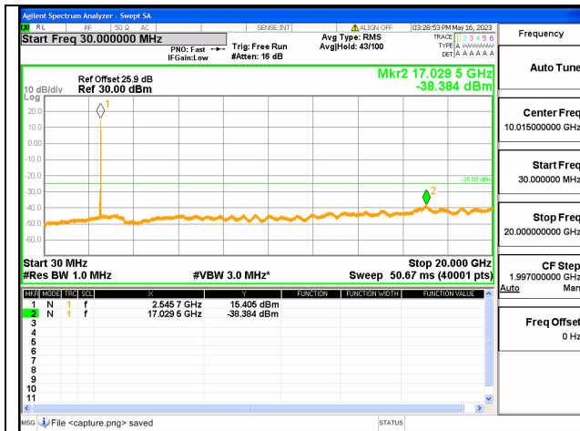
Band7C-30M-20G / 15+10MHz / 1RB+1RB/ QPSK / High CH
