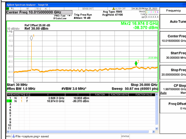
Band41C-30M-20G / 15+10MHz / 75RB+50RB/ QPSK / Low CH
