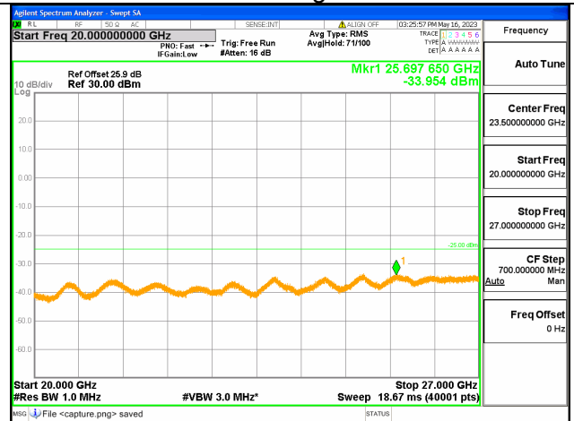
Band7C-20G-27G / 10+20MHz / 1RB+1RB/ QPSK / High CH
