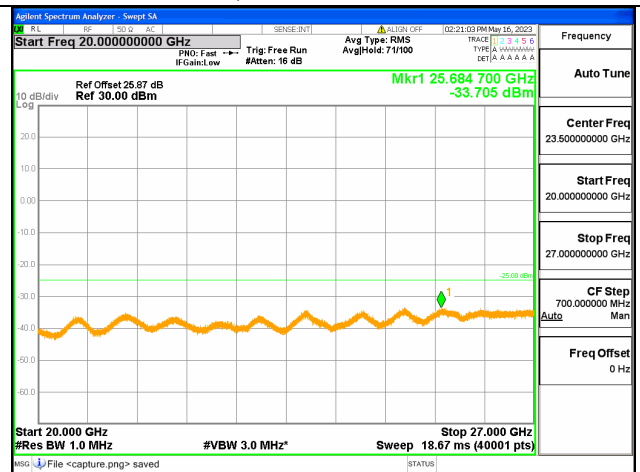
Band7C-20G-27G / 15+20MHz / 1RB+1RB/ QPSK / Low CH
