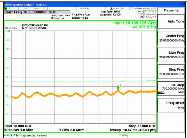
Band7C-20G-27G / 20+15MHz / 100RB+75RB/ QPSK / Low CH
