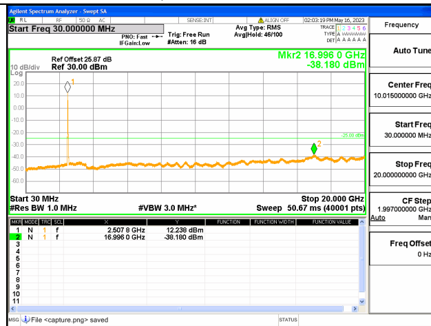
Band7C-30M-20G / 15+15MHz / 75RB+75RB/ QPSK / Low CH
