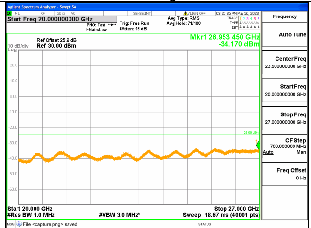
Band7C-20G-27G / 20+10MHz / 1RB+1RB/ QPSK / High CH
