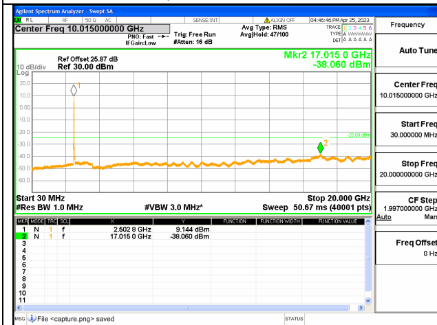
Band41C-30M-20G / 15+20MHz /75RB+100RB/ QPSK / Low CH
