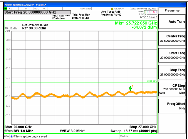
Band7C-20G-27G / 20+15MHz /100RB+75RB/ QPSK / Mid CH
