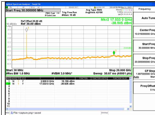
Band7C-30M-20G / 15+10MHz / 1RB+1RB/ QPSK / Low CH
