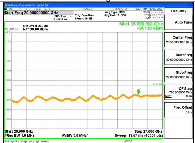
Band7C-20G-27G / 20+15MHz / 100RB+75RB/ QPSK / High CH
