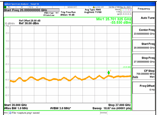
Band7C-20G-27G / 10+20MHz / 50RB+100RB/ QPSK / Mid CH
