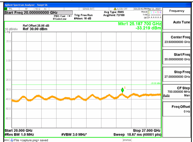
Band7C-20G-27G / 15+10MHz / 75RB+50RB/ QPSK / Low CH
