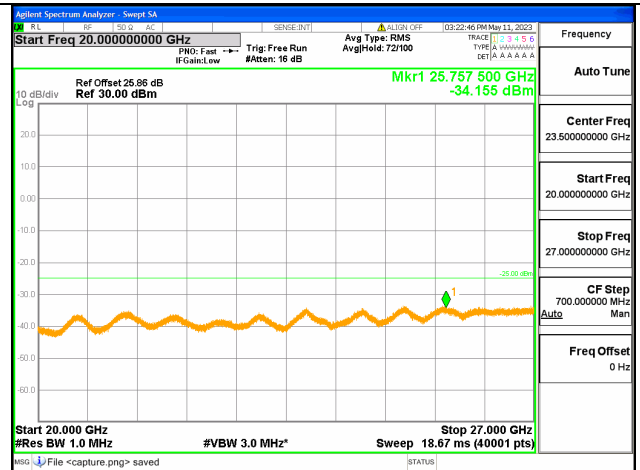
Band7C-20G-27G / 15+10MHz / 1RB+1RB/ QPSK / Low CH
