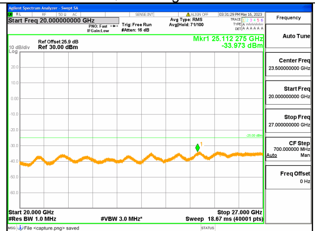
Band7C-20G-27G / 15+15MHz / 75RB+75RB/ QPSK / High CH
