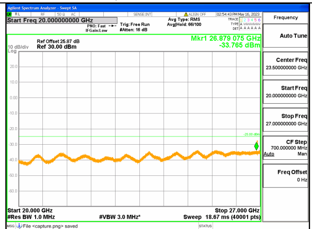
Band7C-20G-27G / 20+20MHz / 100RB+100RB / QPSK / Low CH
