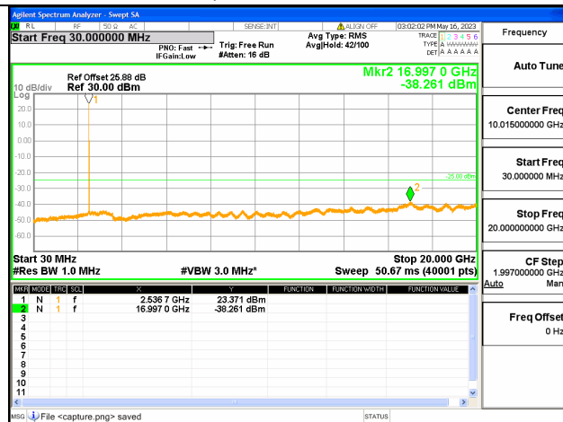
Band7C-30M-20G / 15+10MHz / 1RB+1RB/ QPSK / Mid CH
