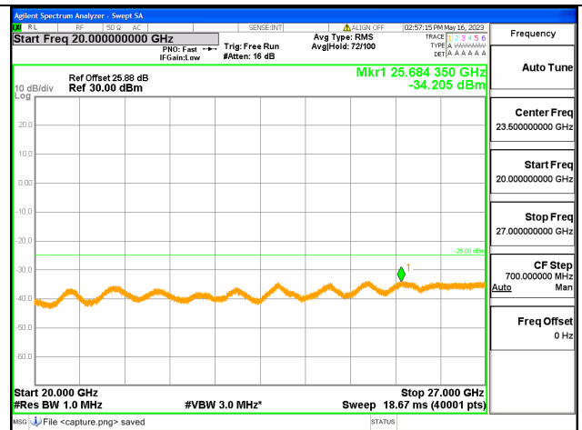
Band7C-20G-27G / 20+10MHz / 1RB+1RB/ QPSK / Mid CH
