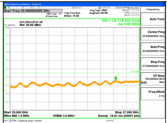
Band7C-20G-27G / 15+15MHz / 75RB+75RB/ QPSK / Low CH
