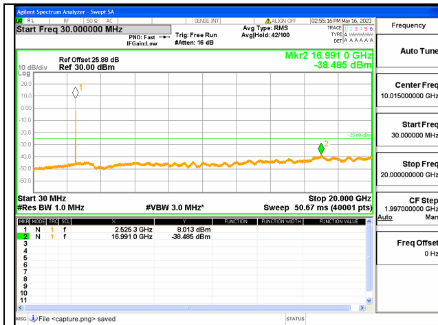
Band7C-30M-20G / 10+20MHz / 1RB+1RB/ QPSK / Mid CH
