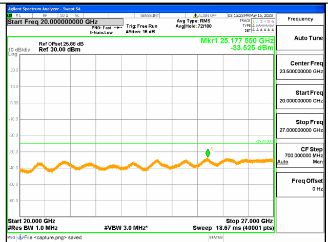
Band7C-20G-27G / 15+20MHz / 1RB+1RB/ QPSK / Mid CH
