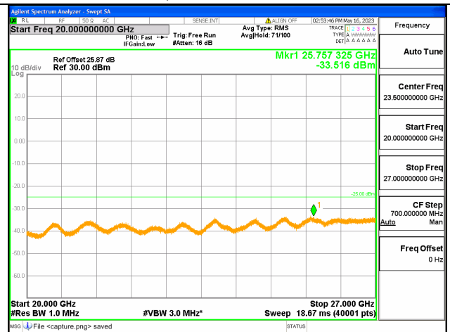
Band7C-20G-27G / 20+20MHz / 1RB+1RB / QPSK / Low CH
