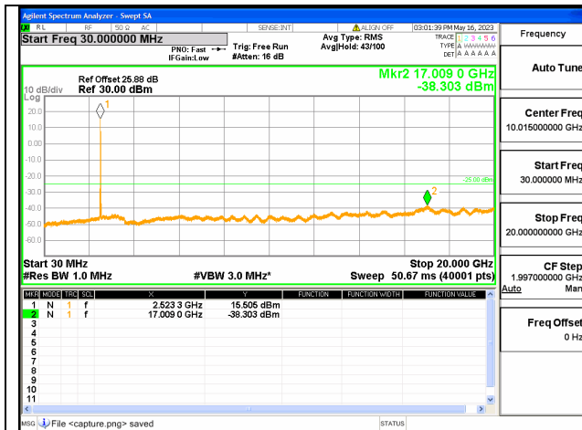
Band7C-30M-20G / 15+10MHz / 1RB+1RB/ QPSK / Mid CH
