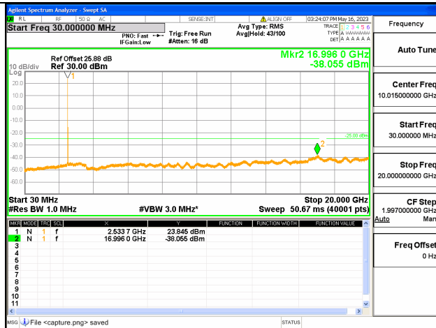
Band7C-30M-20G / 20+20MHz / 1RB+1RB/ QPSK / Mid CH
