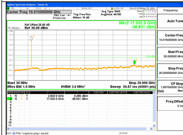
Band41C-30M-20G / 20+10MHz /100RB+50RB/ QPSK / Low CH
