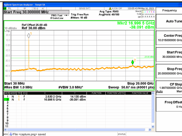
Band7C-30M-20G / 15+10MHz / 75RB+50RB/ QPSK / Mid CH
