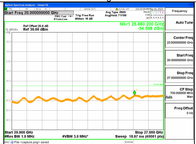
Band7C-20G-27G / 15+20MHz / 75RB+100RB/ QPSK / High CH
