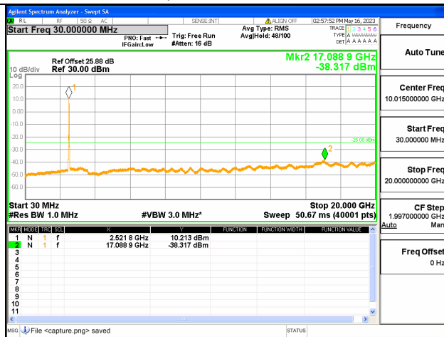
Band7C-30M-20G / 20+10MHz / 100RB+50RB/ QPSK / Mid CH
