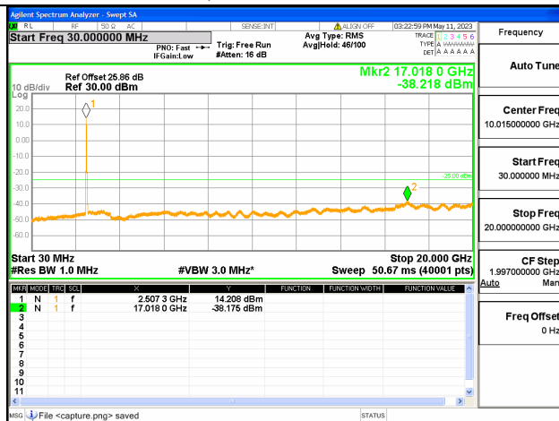
Band7C-30M-20G / 15+10MHz / 75RB+50RB/ QPSK / Low CH
