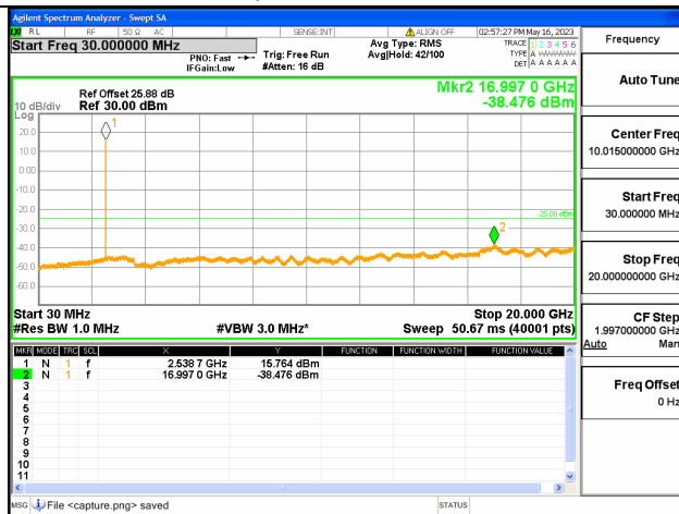
Band7C-30M-20G / 20+10MHz / 1RB+1RB/ QPSK / Mid CH
