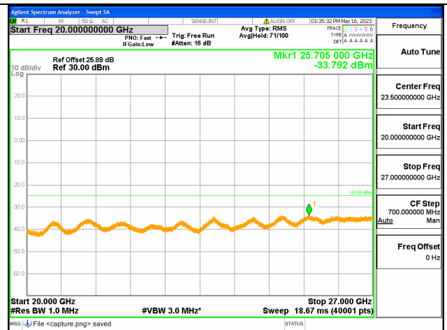
Band7C-20G-27G / 20+20MHz / 1RB+1RB/ QPSK / High CH
