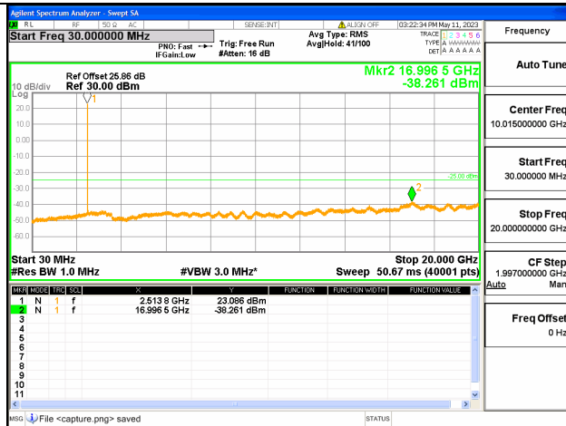
Band7C-30M-20G / 15+10MHz / 1RB+1RB/ QPSK / Low CH
