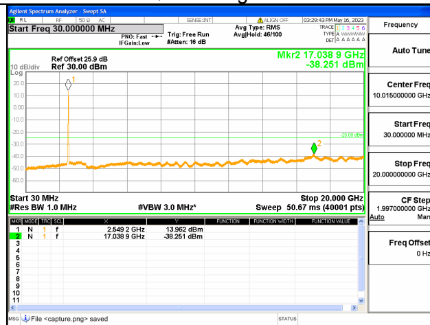
Band7C-30M-20G / 15+10MHz / 75RB+50RB/ QPSK / High CH
