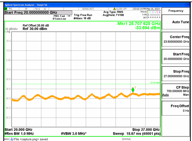
Band7C-20G-27G / 15+10MHz / 1RB+1RB/ QPSK / Mid CH
