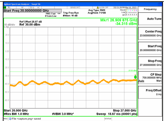
Band7C-20G-27G / 15+20MHz / 75RB+100RB/ QPSK / Low CH
