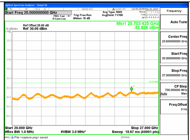
Band7C-20G-27G / 10+20MHz / 1RB+1RB/ QPSK / Mid CH
