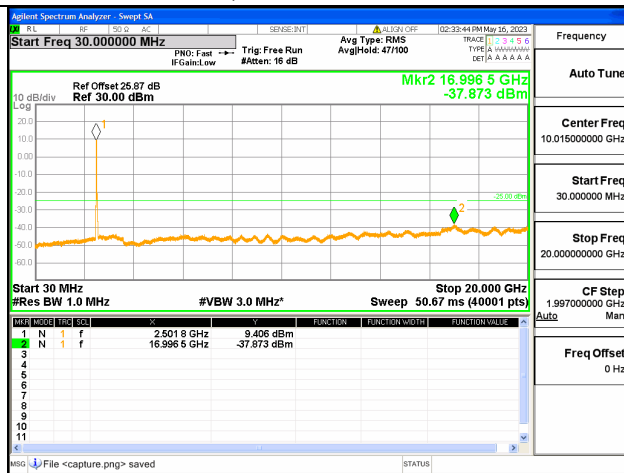
Band7C-30M-20G / 20+15MHz / 100RB+75RB/ QPSK / Low CH
