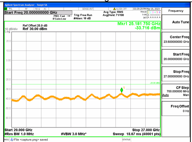
Band7C-20G-27G / 15+10MHz / 1RB+1RB/ QPSK / High CH
