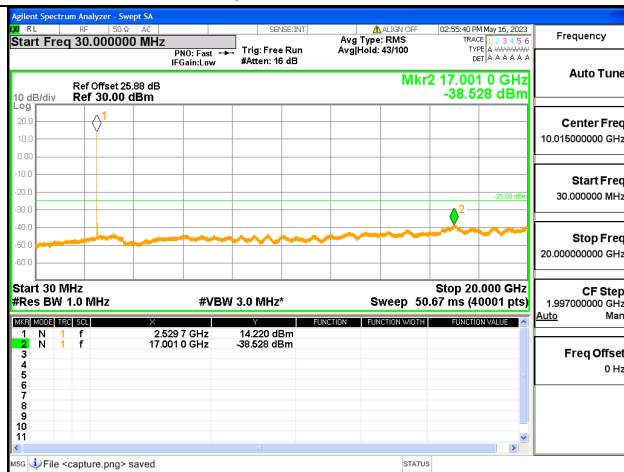
Band7C-30M-20G / 10+20MHz / 1RB+1RB/ QPSK / Mid CH
