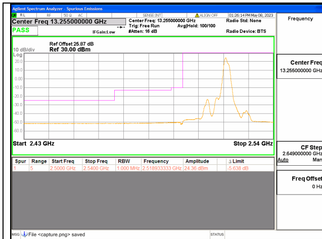
Band7C / 20+10MHz / Low CH / QPSK / 1 RB
