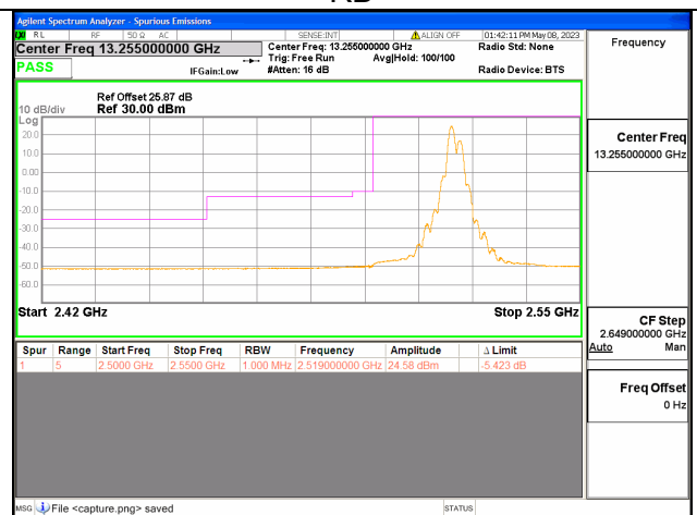
Band7C / 20+20MHz / Low CH / QPSK / 1 RB
