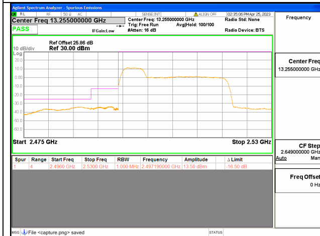
Band41C / 5+20MHz / Low CH / QPSK / 25 RB
