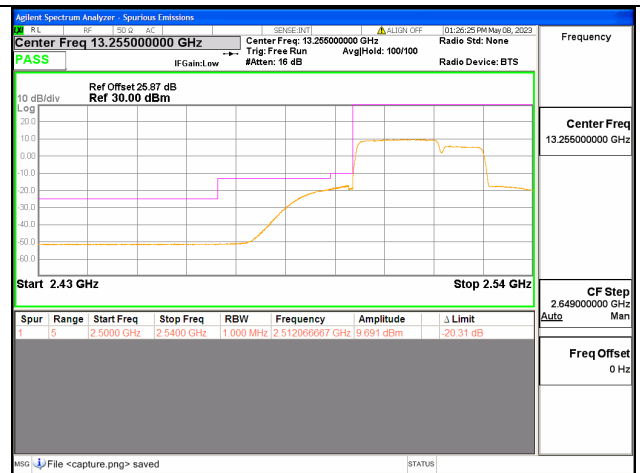
Band7C / 20+10MHz / Low CH / QPSK / 100 RB
