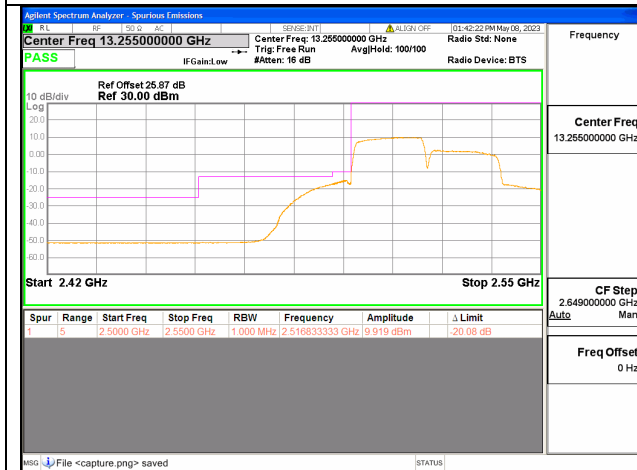
Band7C / 20+20MHz / Low CH / QPSK / 100 RB
