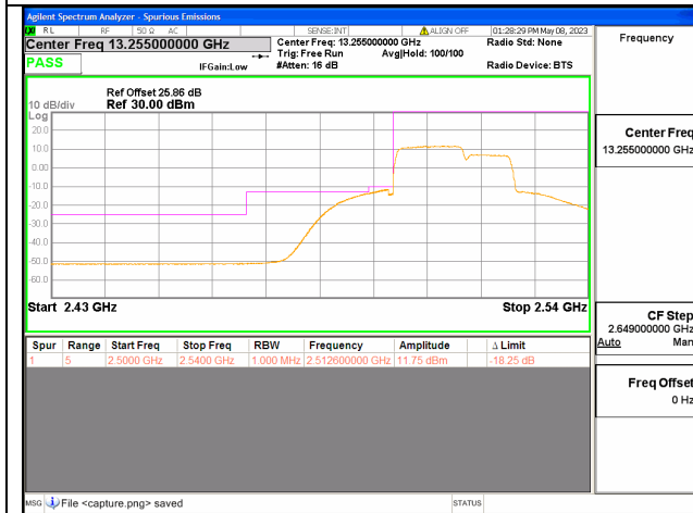
Band7C / 15+10MHz / Low CH / QPSK / 75 RB
