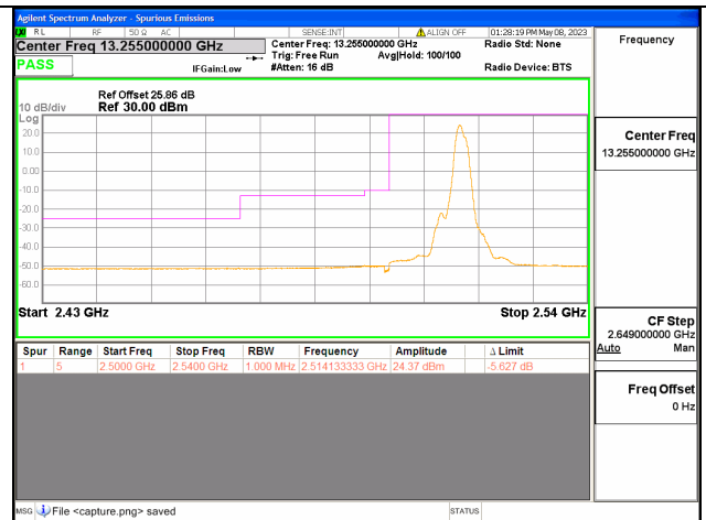
Band7C / 15+10MHz / Low CH / QPSK / 1 RB
