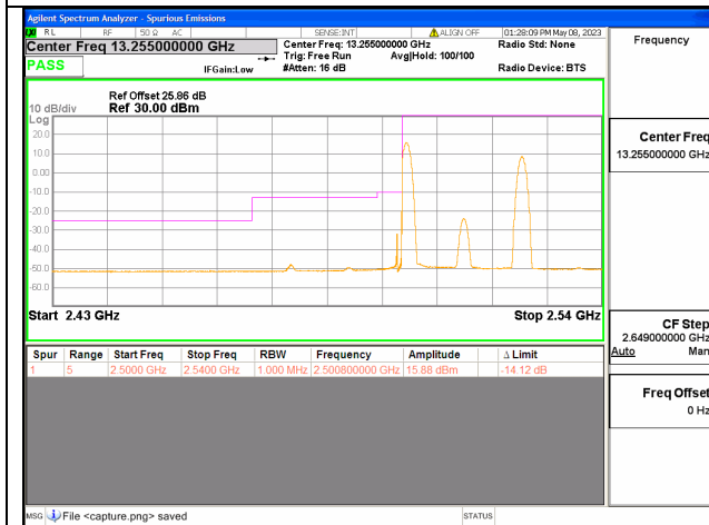
Band7C / 15+10MHz / Low CH / QPSK / 1 RB
