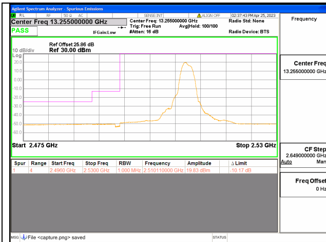
Band41C / 15+10MHz / Low CH / QPSK / 1 RB
