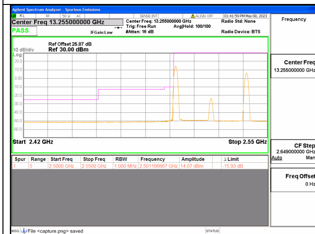
Band7C / 20+20MHz / Low CH / QPSK / 1 RB
