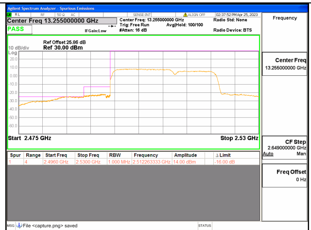
Band41C / 15+10MHz / Low CH / QPSK / 75 RB
