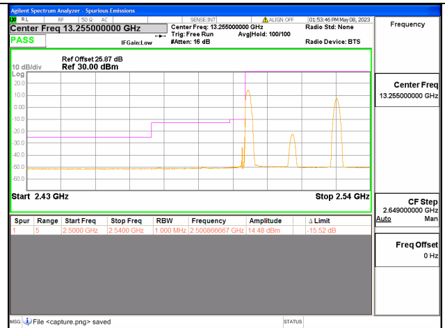
Band7C / 15+15MHz / Low CH / QPSK / 1 RB
