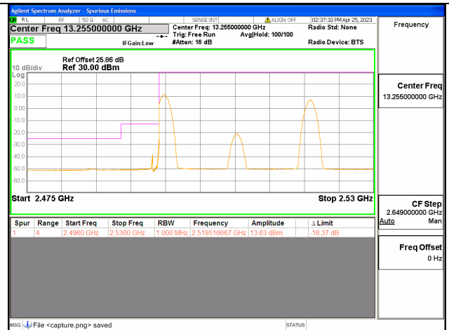
Band41C / 15+10MHz / Low CH / QPSK / 1 RB
