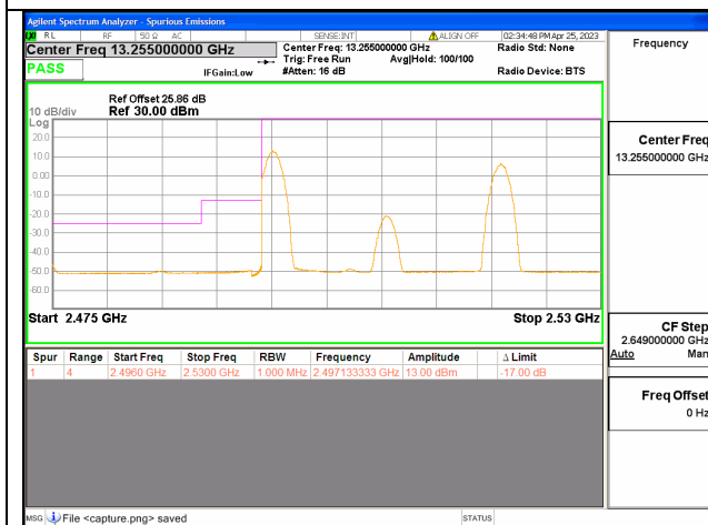
Band41C / 5+20MHz / Low CH / QPSK / 1 RB
