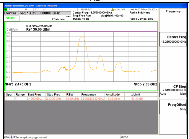
Band41C / 5+20MHz / Low CH / QPSK / 1 RB
