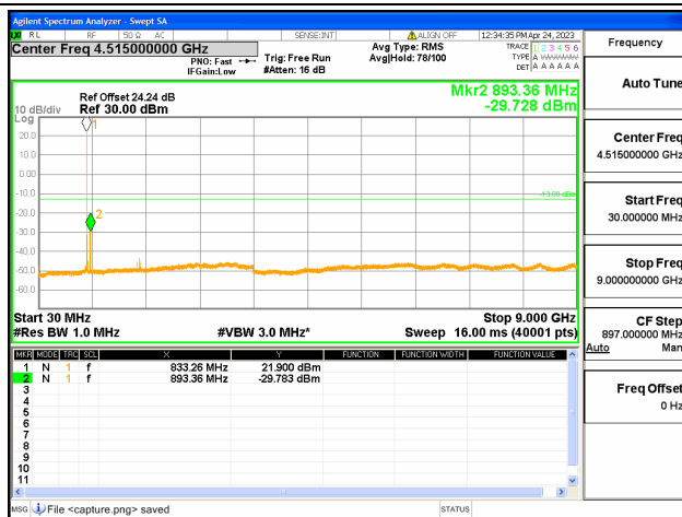
Band19 / 10MHz / Mid CH / QPSK
