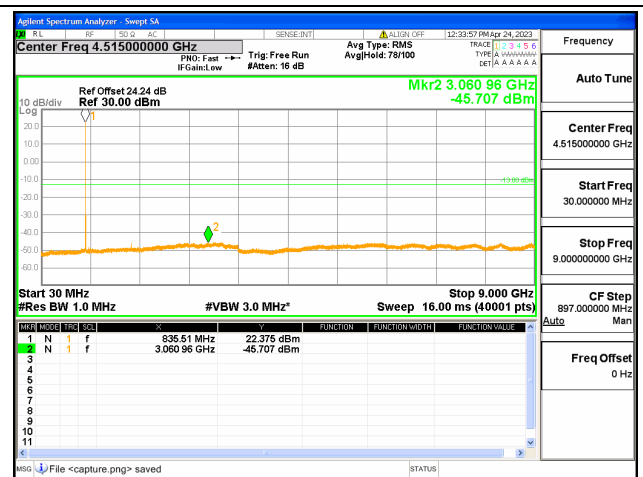
Band19 / 5MHz / Mid CH / QPSK
