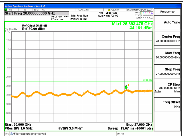
Band41-20G-27G / 5MHz / Low CH / QPSK
