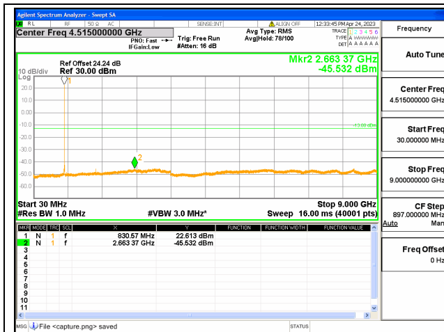
Band19 / 5MHz / Low CH / QPSK
