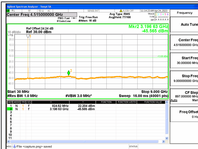
Band18 part22 / 5MHz / Low CH / QPSK
