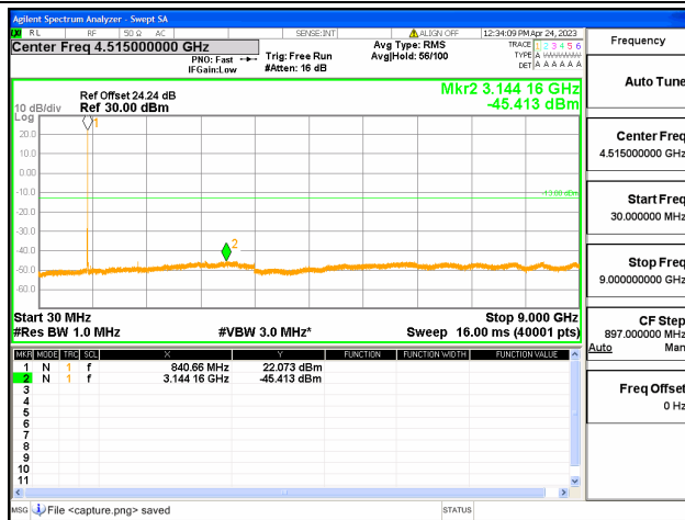
Band19 / 5MHz / High CH / QPSK
