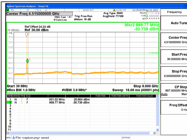
Band19 / 15MHz / Low CH / QPSK
