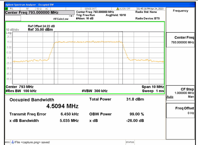
Band14 / 5MHz / QPSK/ Mid CH
