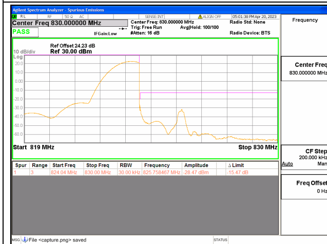
Band18 part90 / 5MHz / High CH / QPSK / 1 RB
