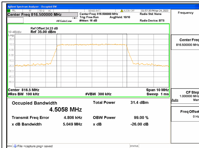
Band26 Part90 / 5MHz / QPSK/ Low CH
