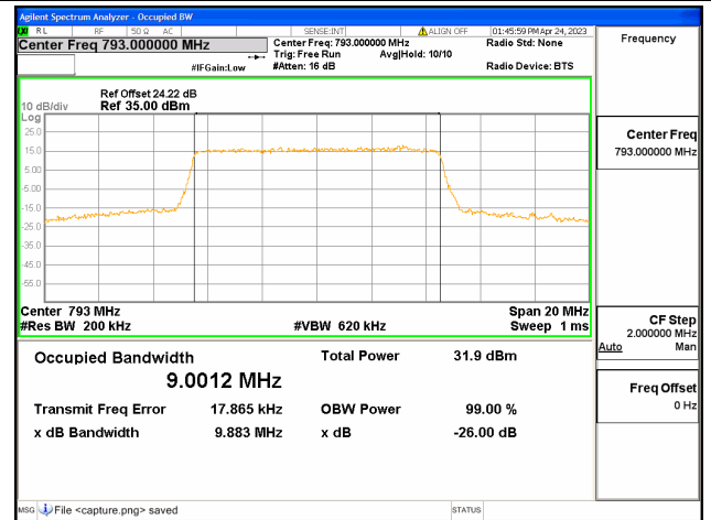
Band14 / 10MHz / QPSK/ Mid CH
