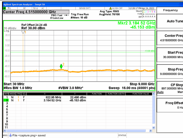
Band26 Part90 / 1.4MHz / High CH / QPSK
