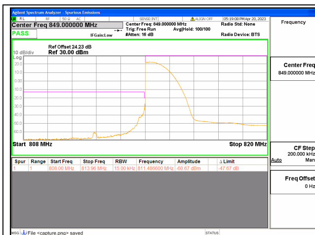
Band26 Part90 / 1.4MHz / Low CH / QPSK / 1 RB
