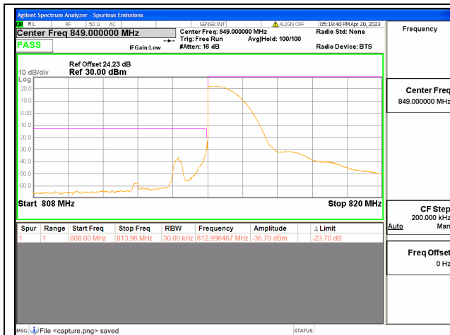
Band26 Part90 / 3MHz / Low CH / QPSK / 1 RB
