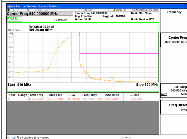
Band26 Part90 / 1.4MHz / High CH / QPSK / 1 RB
