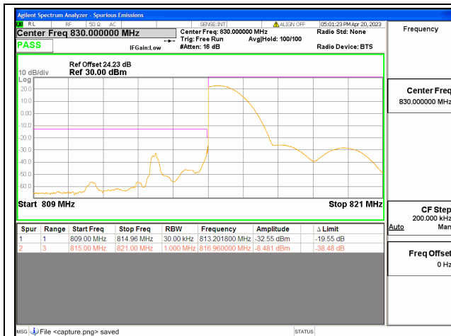
Band18 part90 / 5MHz / Low CH / QPSK / 1 RB
