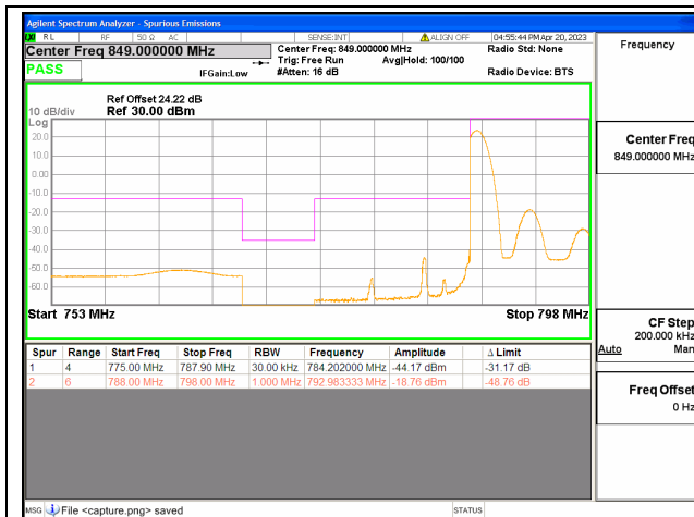
Band14 / 10MHz / Low CH / QPSK / 1 RB
