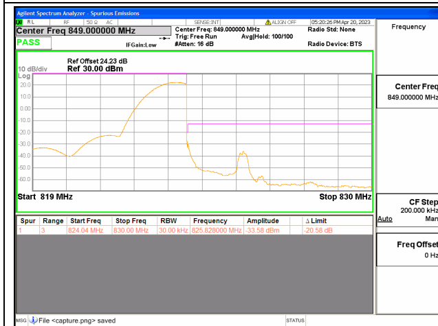
Band26 Part90 / 5MHz / High CH / QPSK / 1 RB
