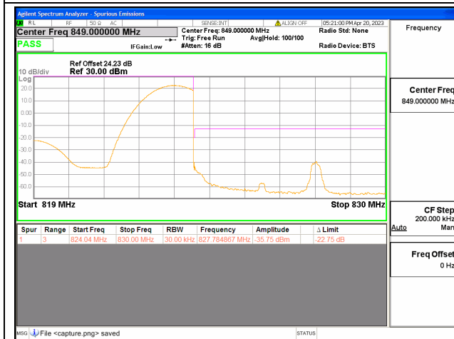
Band26 Part90 / 10MHz / High CH / QPSK / 1 RB
