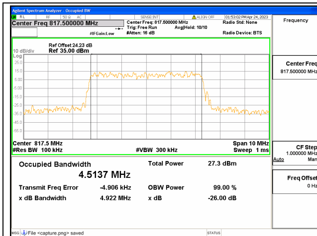
Band18 part90 / 5MHz / QPSK/ Low CH
