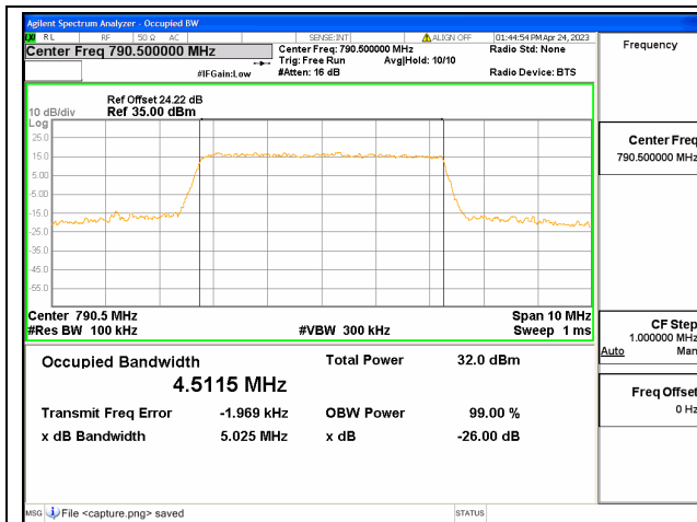
Band14 / 5MHz / QPSK/ Low CH
