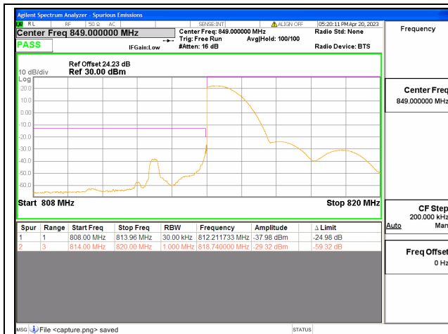
Band26 Part90 / 5MHz / Low CH / QPSK / 1 RB
