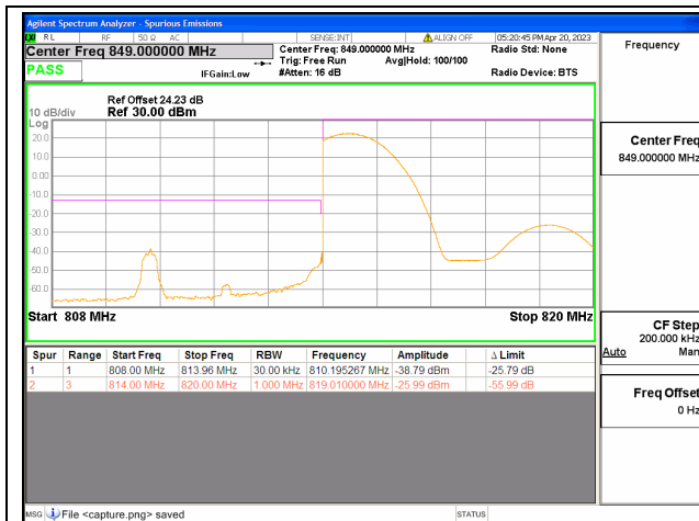
Band26 Part90 / 10MHz / Low CH / QPSK / 1 RB
