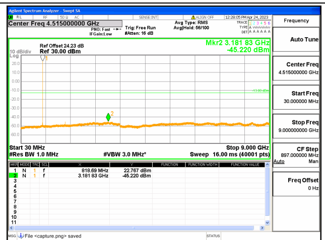
Band26 Part90 / 1.4MHz / Mid CH / QPSK
