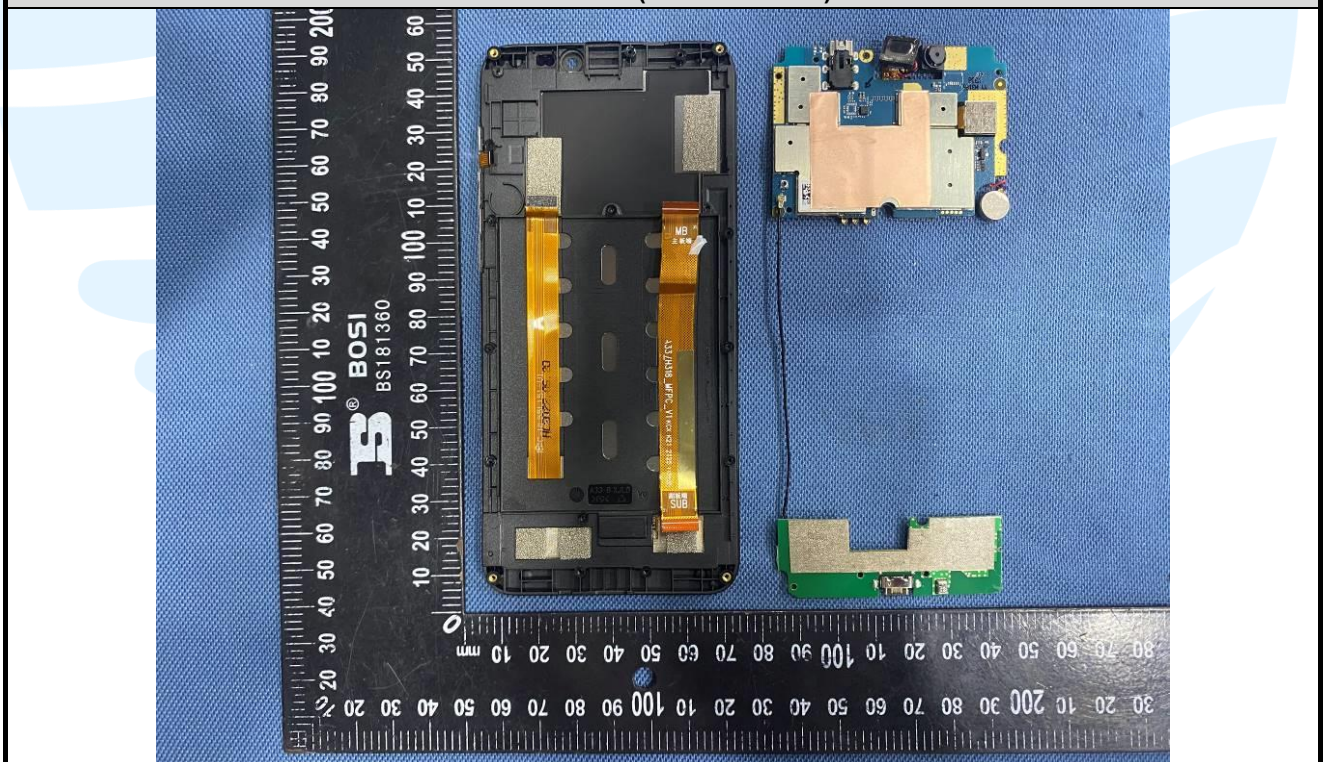
EUT Photo (LCD Module 1)
