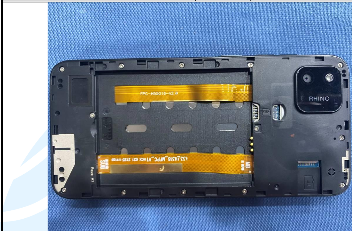
EUT Photo (LCD Module 2)
