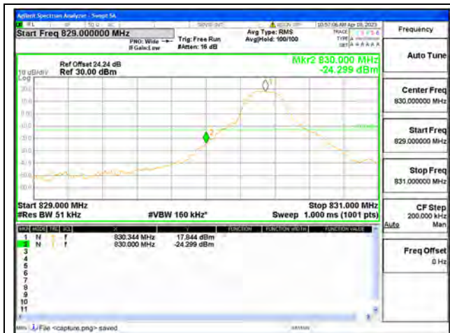
Band19 / 5MHz / Low CH / QPSK / 1 RB
