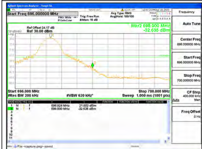
Band71 / 20MHz / High CH / QPSK / 1 RB
