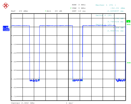
DH5
