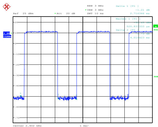
2-DH5
