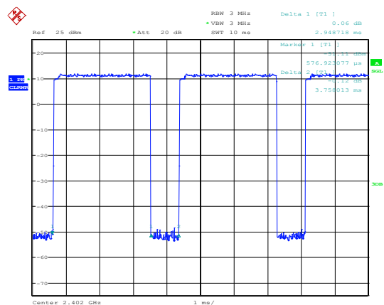
3-DH5
