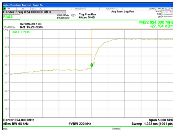
B5_HSDPA_Lower_Band edge
