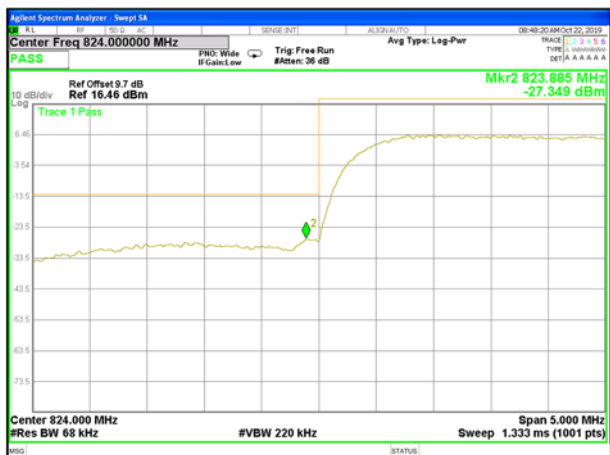
B5_WCDMA_Lower_Band edge
