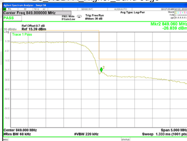
B5_HSUPA_Higher_Band edge
