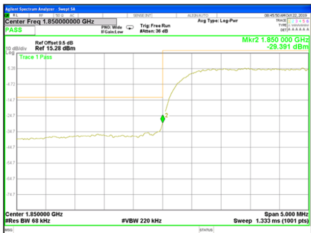
B2_WCDMA_Lower_Band edge
