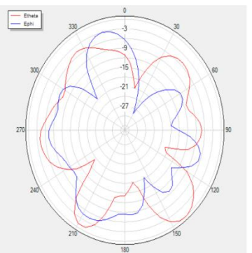
V Phi=0 freq=2500MHz
