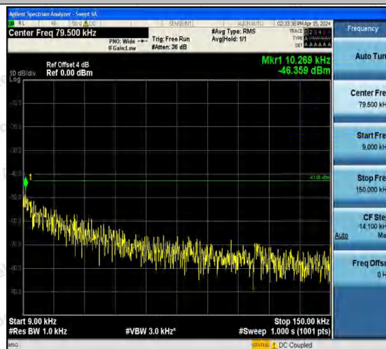
Band4-1513-5-0.009~0.15MHz-PASS
