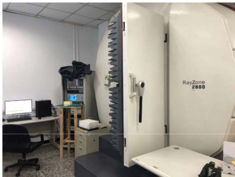
Auden GTS2800 ↑
