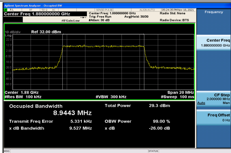
Band2-10MHz-QPSK-18900-50RB#0-8.9443
