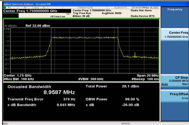
Band4-10MHz-QPSK-20350-50RB#0-8.9587
