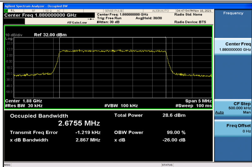
Band2-3MHz-QPSK-18900-15RB#0-2.6755
