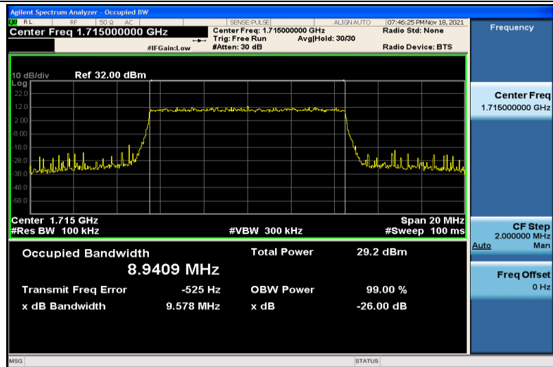
Band4-10MHz-QPSK-20000-50RB#0-8.9409
