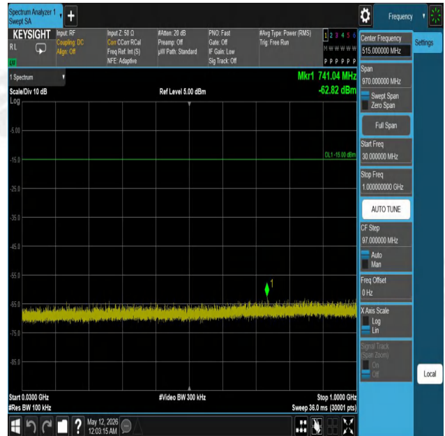
11G-Ant1-2437-30~1000-PASS
