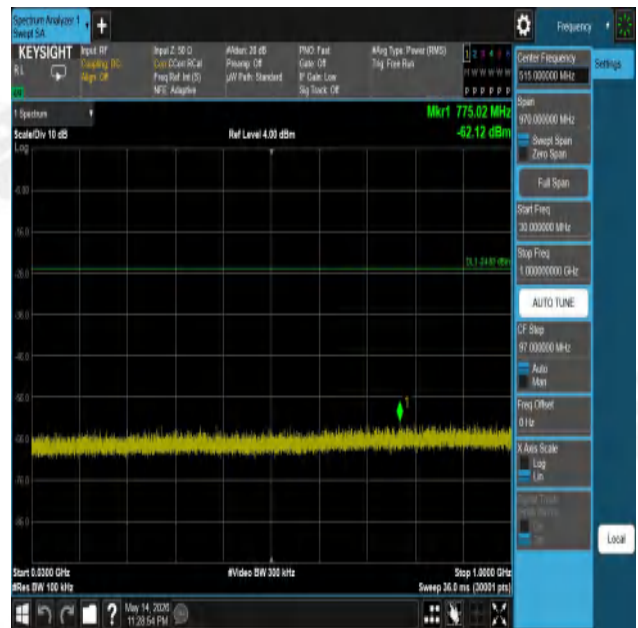
11G-Ant1-2437-30~1000-PASS
