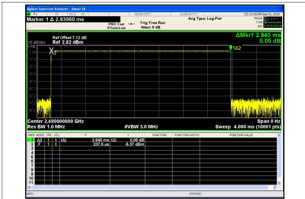
(DH5_2480M, GFSK)
