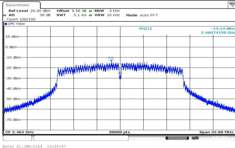
11N20SISO-Ant1-2462--14.14-0.00-0.00-0.00
