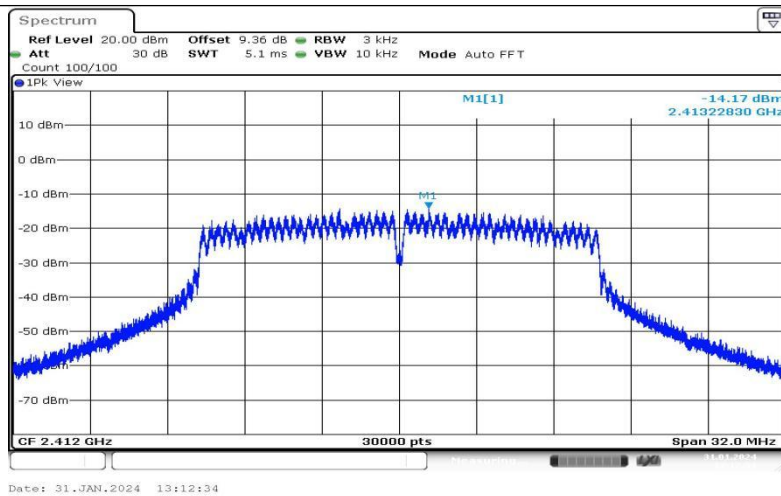
11G-Ant1-2412--14.17-0.00-0.00-0.00
