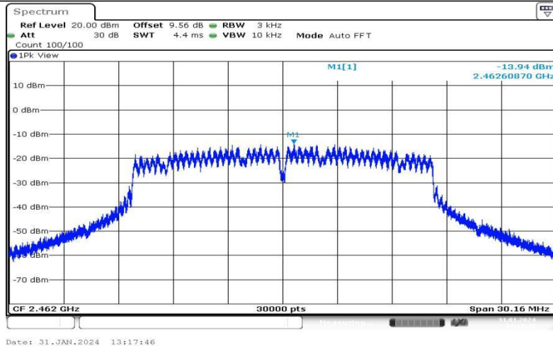
11G-Ant1-2462--13.94-0.00-0.00-0.00
