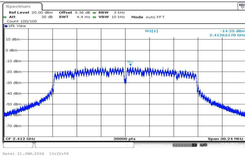
11N20SISO-Ant1-2412--14.25-0.00-0.00-0.00
