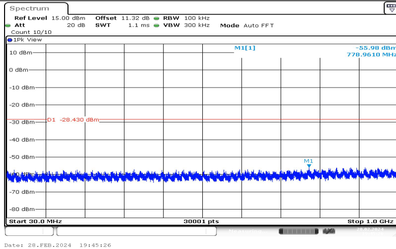
3DH5-Ant1-2480-30~1000--8.43
