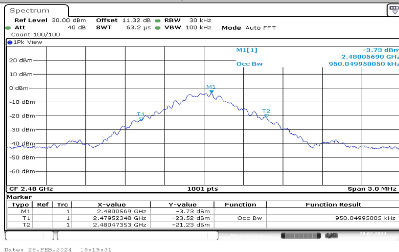
DH5-Ant1-2480
