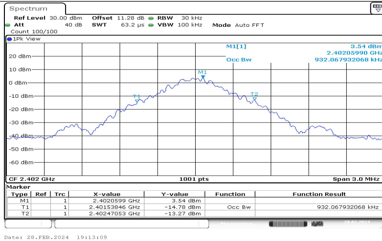
DH5-Ant1-2402
