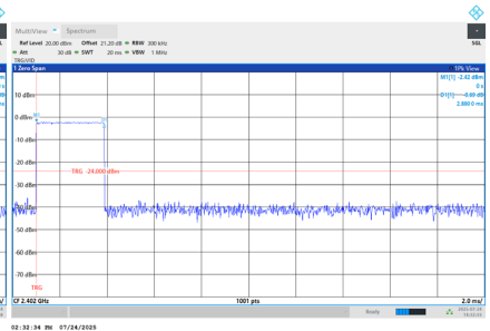
DH5
