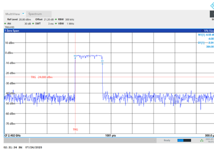
DH1
