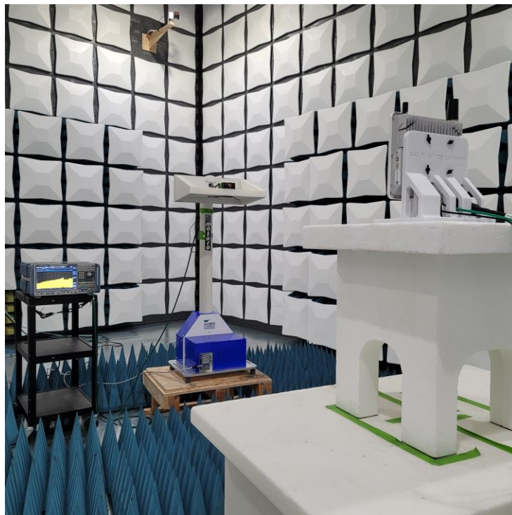
Setup 8. Test Setup >40GHz - DU
