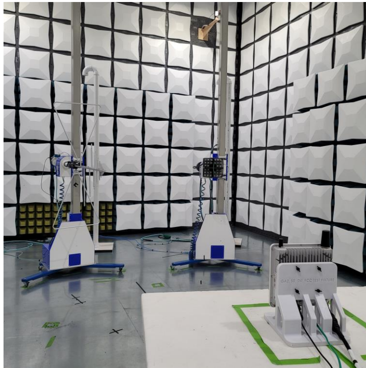
Setup 2. Test Setup <1GHz - DU
