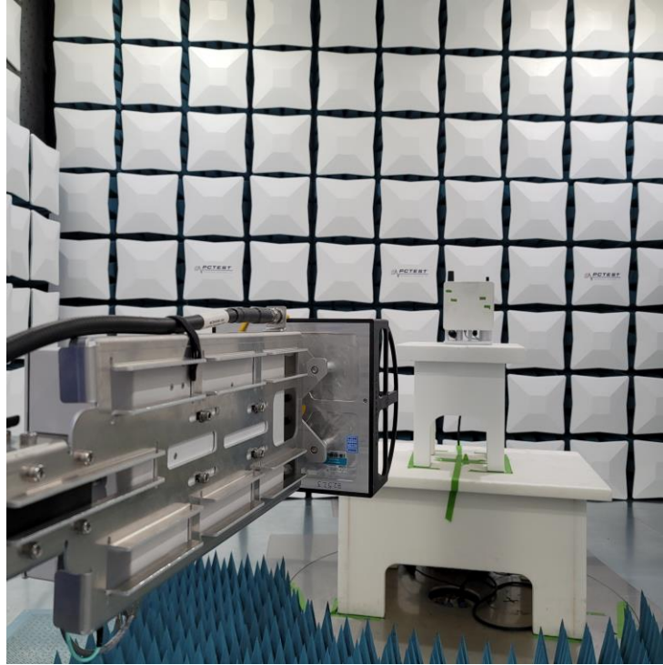
Setup 3. Test Setup 1-18GHz - DU
