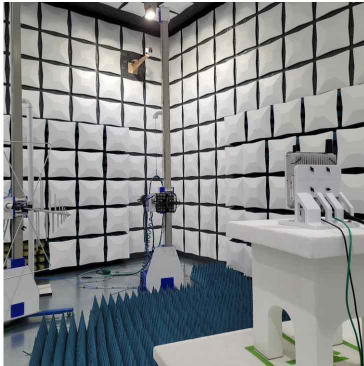
Setup 4. Test Setup 1-18GHz - DU
