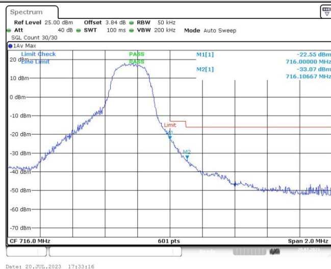
Band12-3MHz-QPSK-23165-15RB#0
