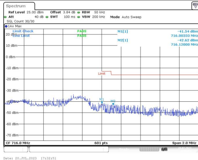
Band12-3MHz-QPSK-23165-1RB#14
