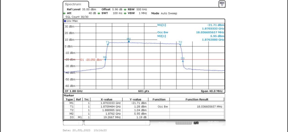
Band2-20MHz-QPSK-19100-100RB#0
