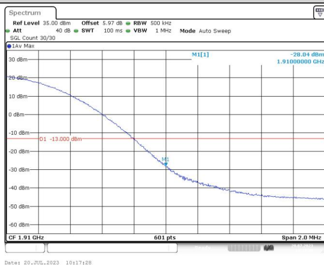
Band2-20MHz-QPSK-19100-100RB#0
