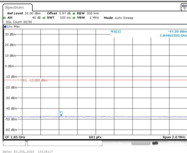
Band2-20MHz-16QAM-18700-100RB#0
