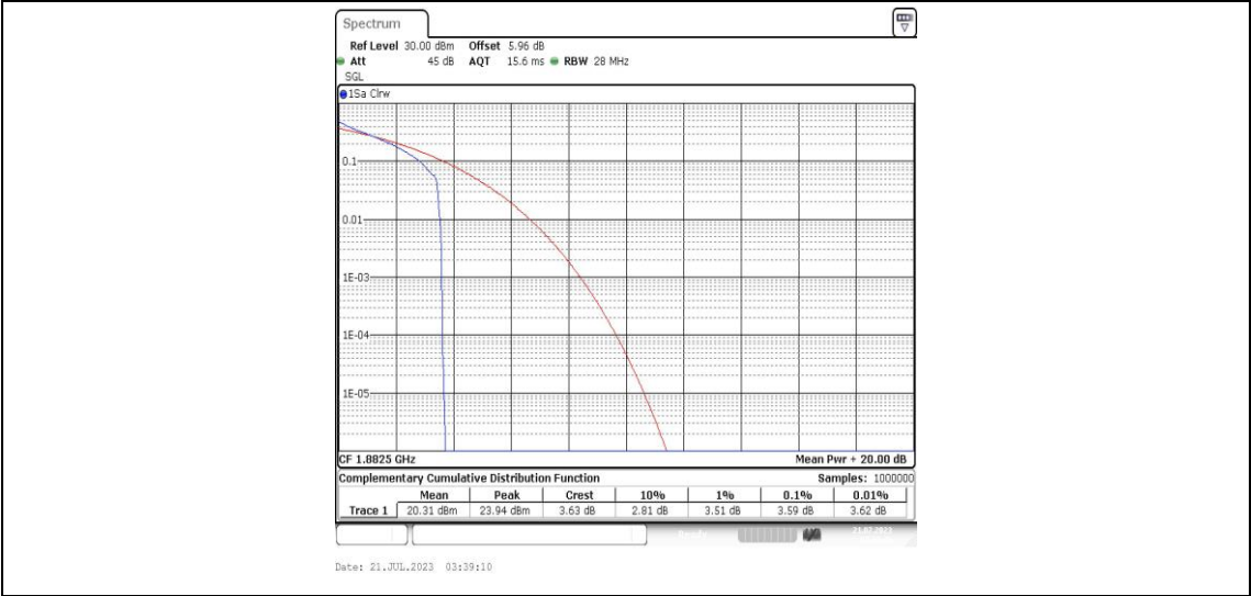
Band25-20MHz-QPSK-26365-1RB#0-PASS
