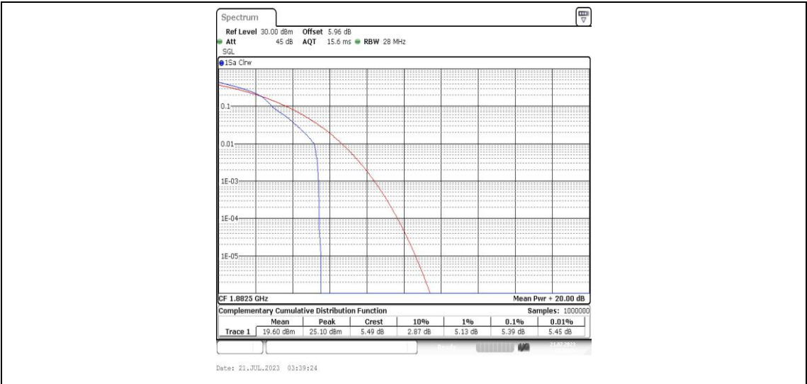
Band25-20MHz-16QAM-26365-1RB#0-PASS
