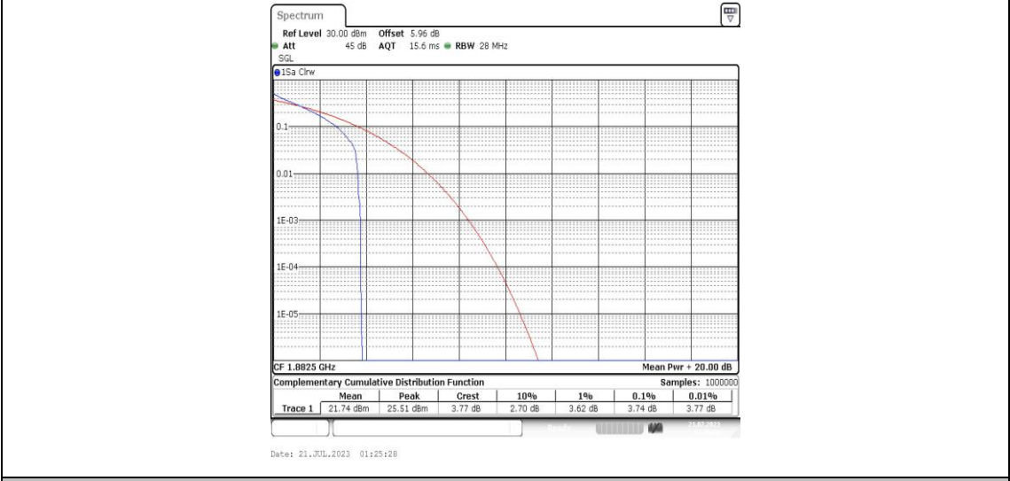
Band25-3MHz-QPSK-26365-1RB#0-PASS
