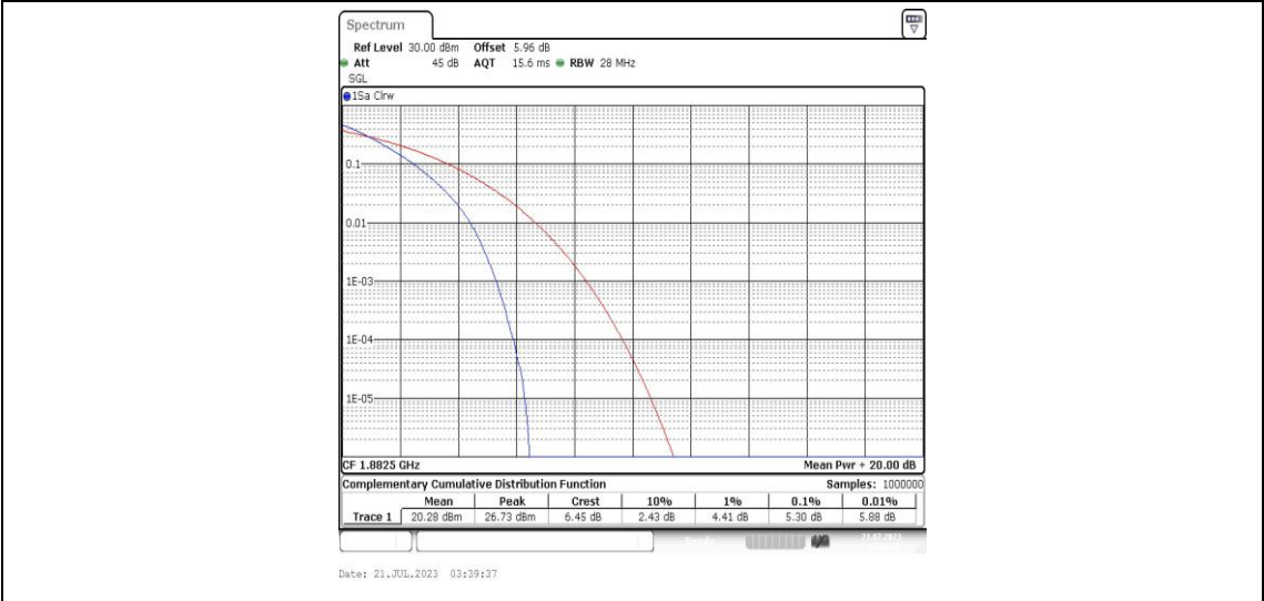
Band25-20MHz-QPSK-26365-100RB#0-PASS
