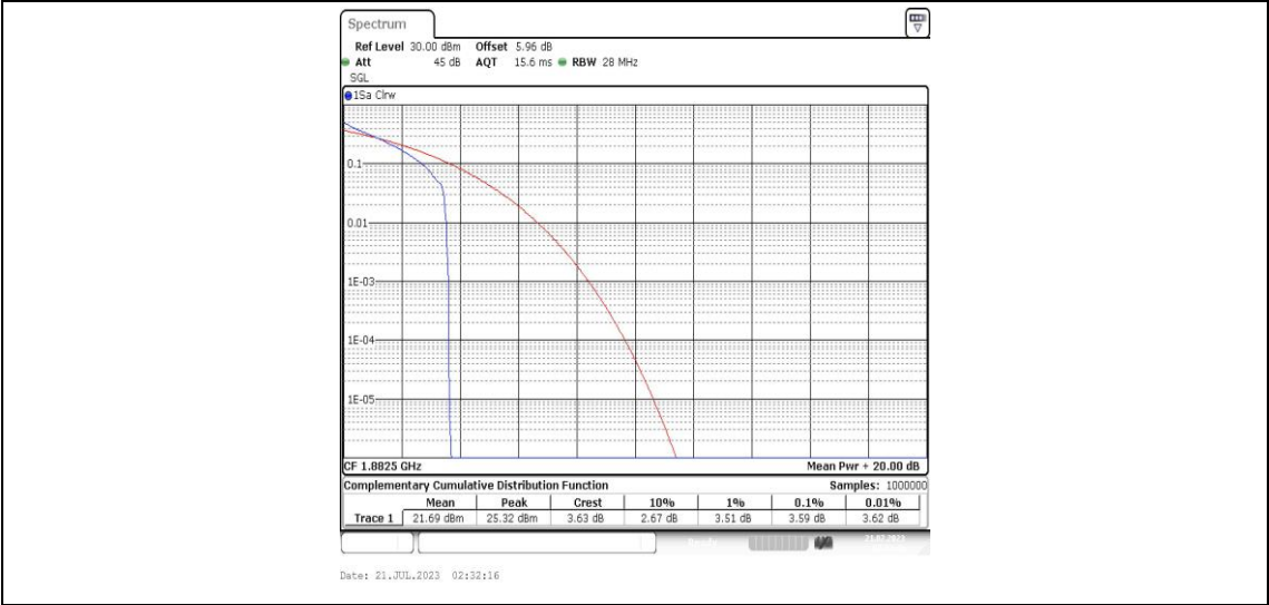
Band25-10MHz-QPSK-26365-1RB#0-PASS
