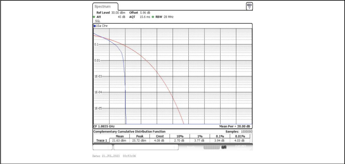
Band25-1.4MHz-QPSK-26365-1RB#0-PASS
