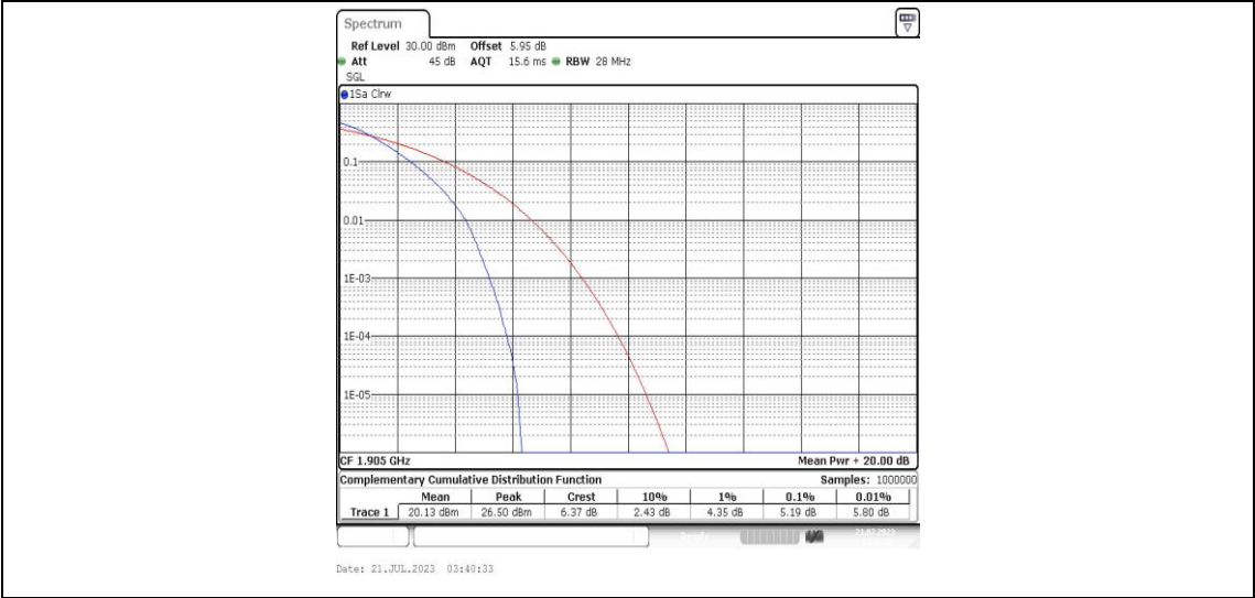
Band25-20MHz-QPSK-26590-100RB#0-PASS
