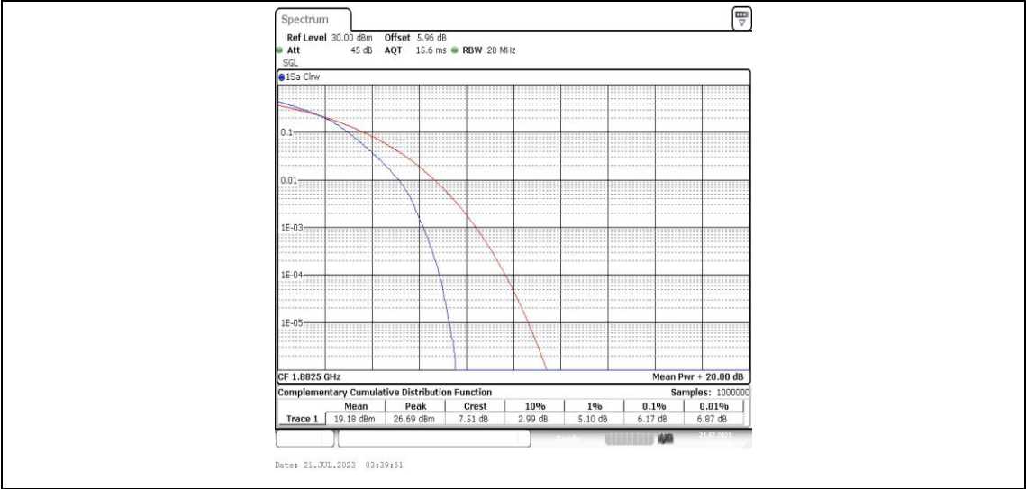
Band25-20MHz-16QAM-26365-100RB#0-PASS
