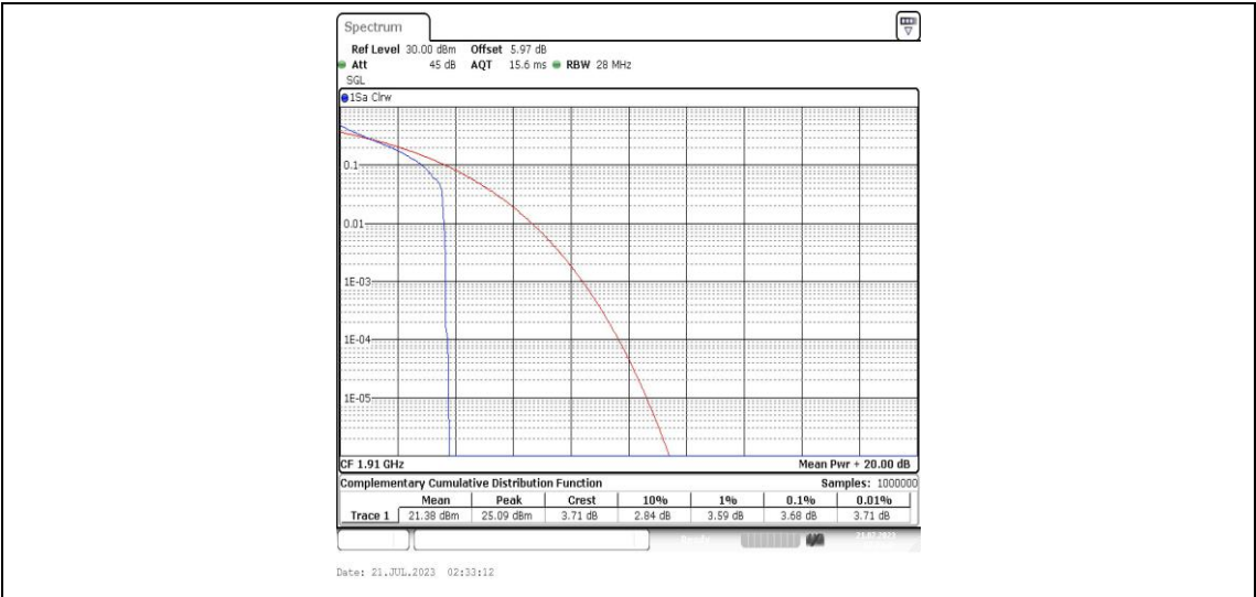
Band25-10MHz-QPSK-26640-1RB#0-PASS
