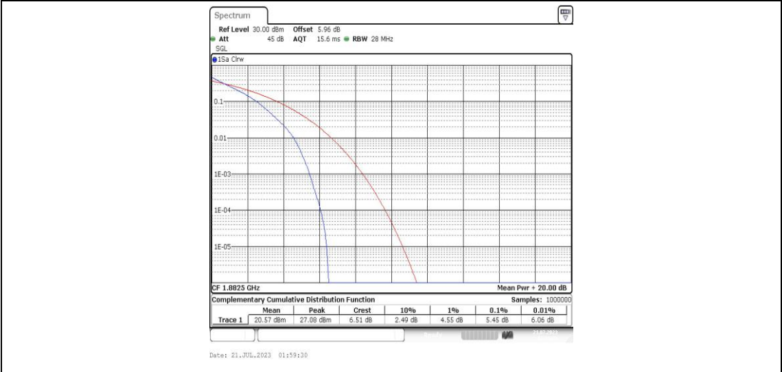
Band25-5MHz-QPSK-26365-25RB#0-PASS
