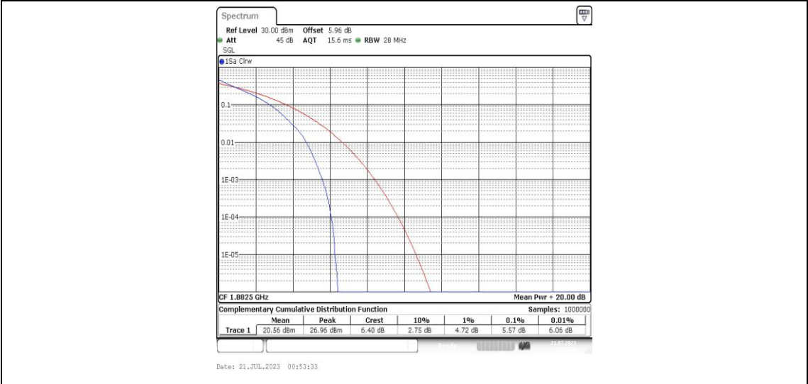
Band25-1.4MHz-QPSK-26365-6RB#0-PASS
