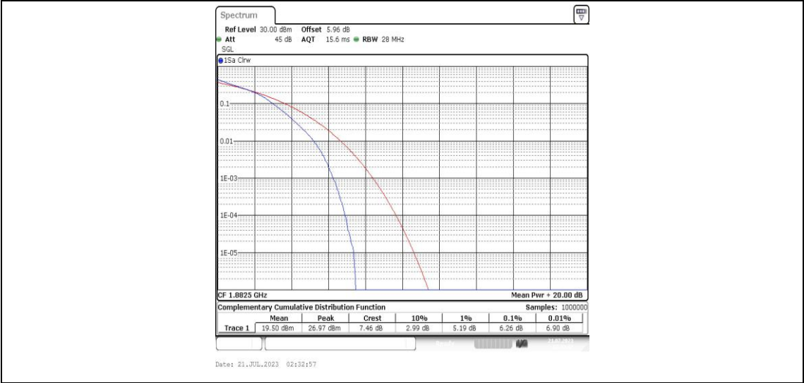
Band25-10MHz-16QAM-26365-50RB#0-PASS
