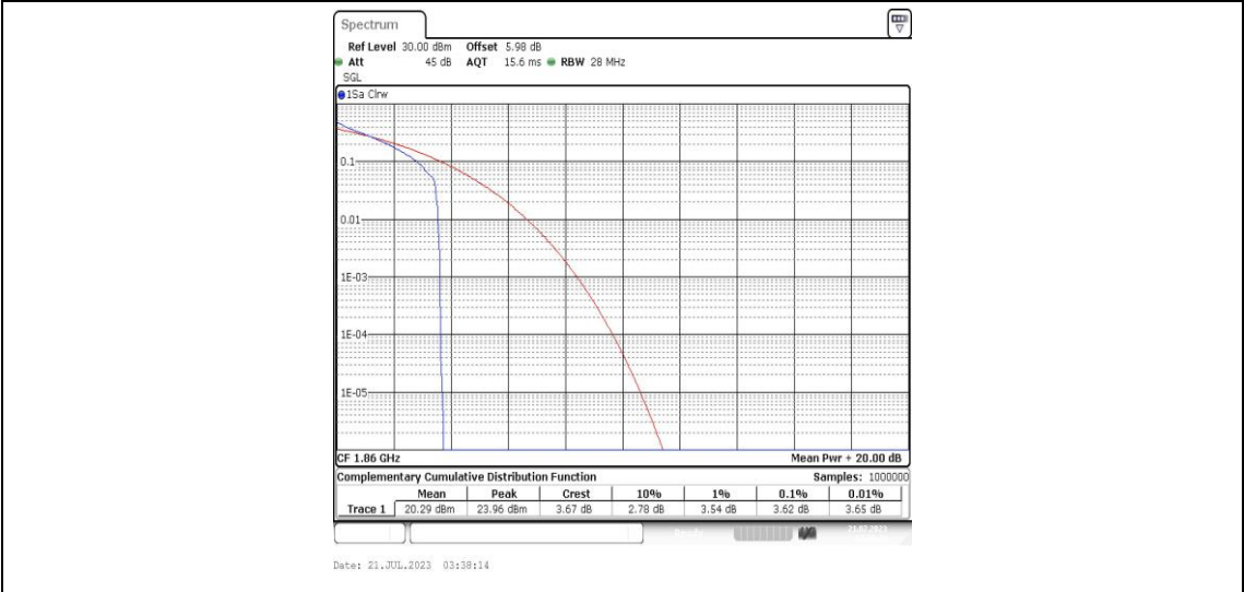
Band25-20MHz-QPSK-26140-1RB#0-PASS
