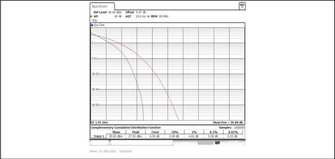
Band25-10MHz-QPSK-26640-50RB#0-PASS
