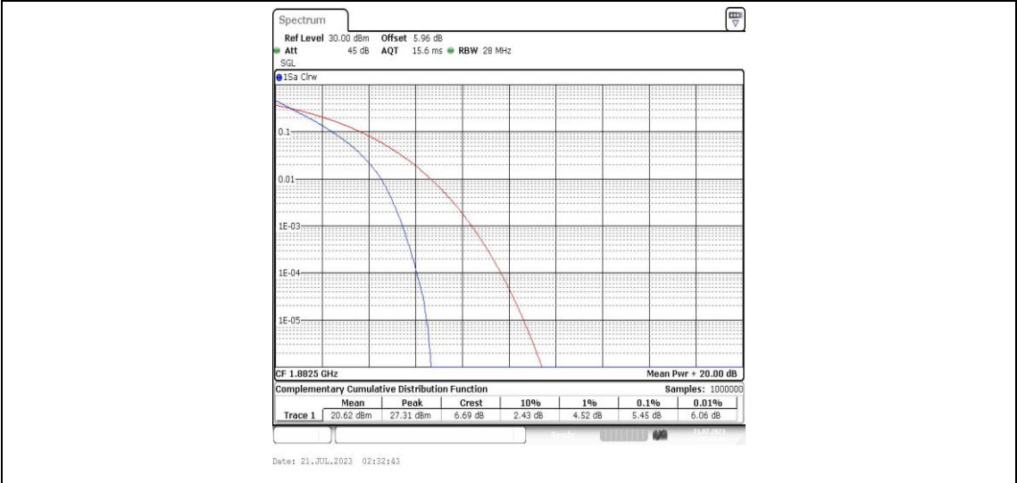
Band25-10MHz-QPSK-26365-50RB#0-PASS
