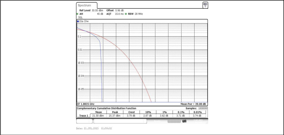
Band25-5MHz-QPSK-26365-1RB#0-PASS
