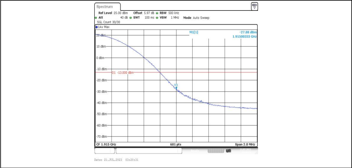
Band25-20MHz-QPSK-26590-1RB#99-PASS
