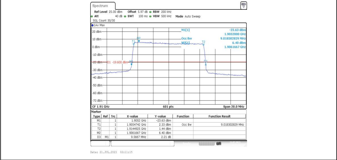
Band25-10MHz-QPSK-26640-50RB#0-PASS
