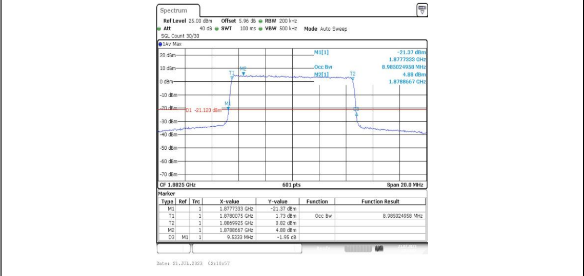
Band25-10MHz-16QAM-26365-50RB#0-PASS
