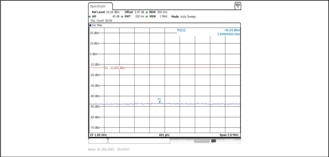
Band25-20MHz-QPSK-26140-1RB#99-PASS
