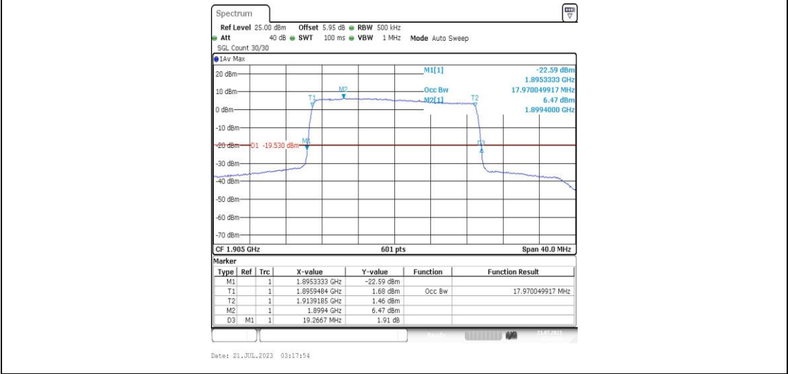
Band25-20MHz-QPSK-26590-100RB#0-PASS
