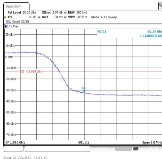
Band25-10MHz-QPSK-26640-50RB#0-PASS
