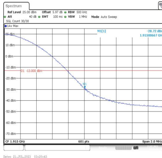
Band25-20MHz-16QAM-26590-1RB#99-PASS
