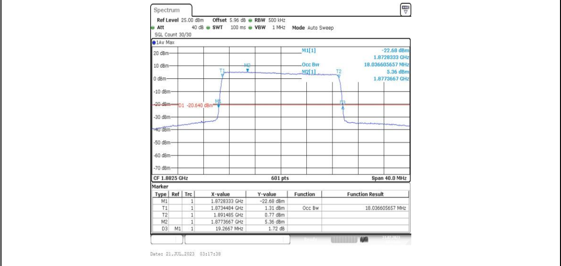
Band25-20MHz-16QAM-26365-100RB#0-PASS
