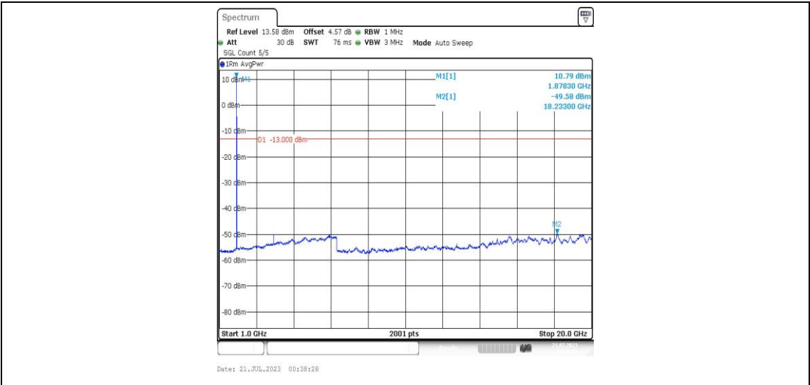
Band25-1.4MHz-QPSK-26365-1RB#0-Range4:1000~20000MHz-PASS
