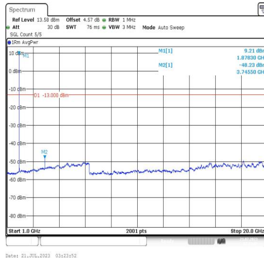
Band25-20MHz-QPSK-26365-1RB#0-Range4:1000~20000MHz-PASS
