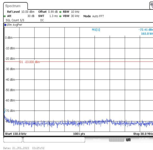
Band25-20MHz-16QAM-26590-1RB#0-Range2:0.15~30MHz-PASS
