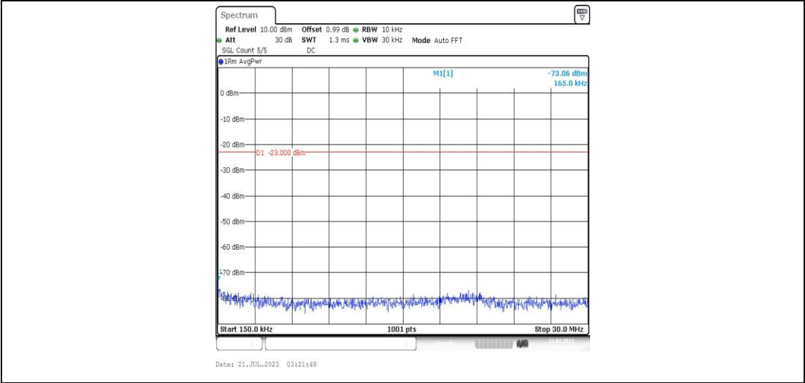
Band25-20MHz-QPSK-26140-1RB#0-Range2:0.15~30MHz-PASS
