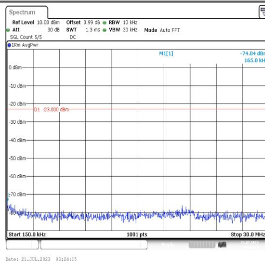
Band25-20MHz-16QAM-26365-1RB#0-Range2:0.15~30MHz-PASS
