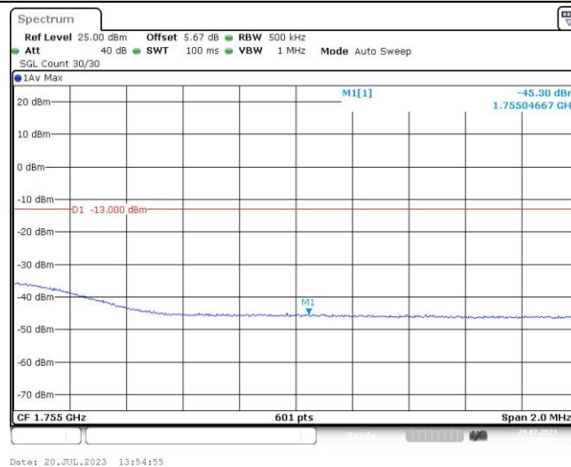
Band4-20MHz-QPSK-20300-1RB#99
