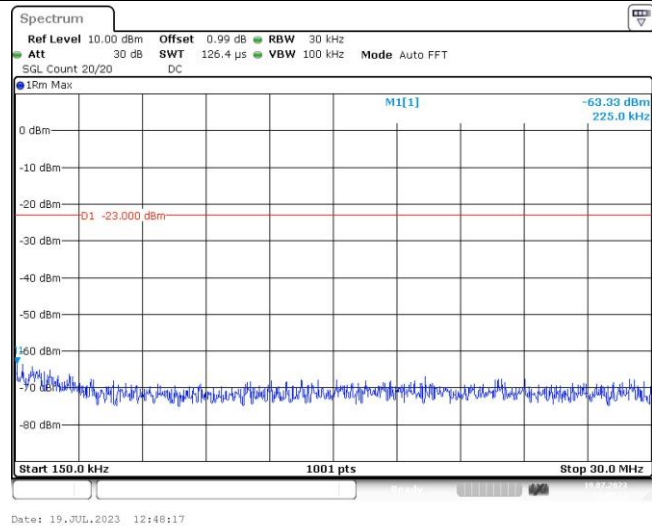
Band2-9262-3-30~1000MHz
