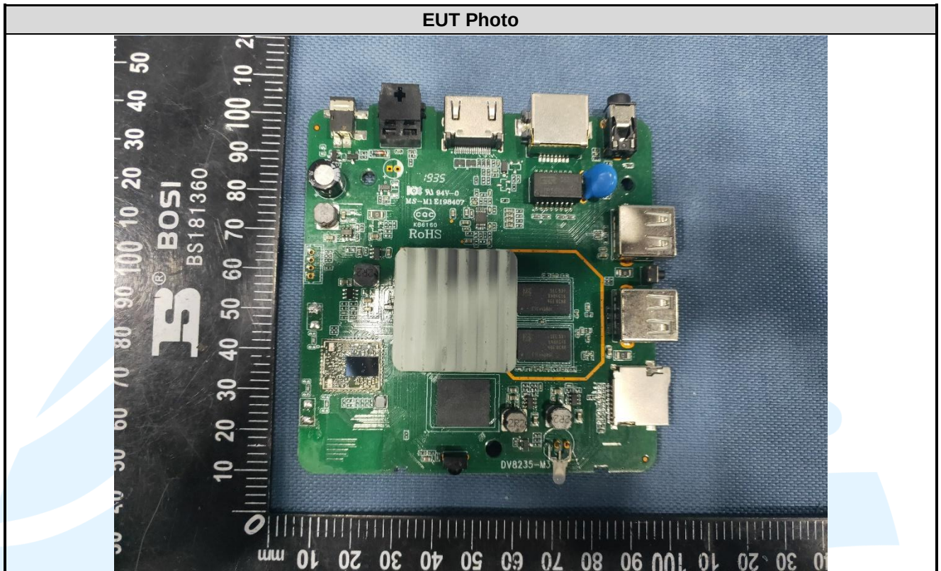
EUT Photo
