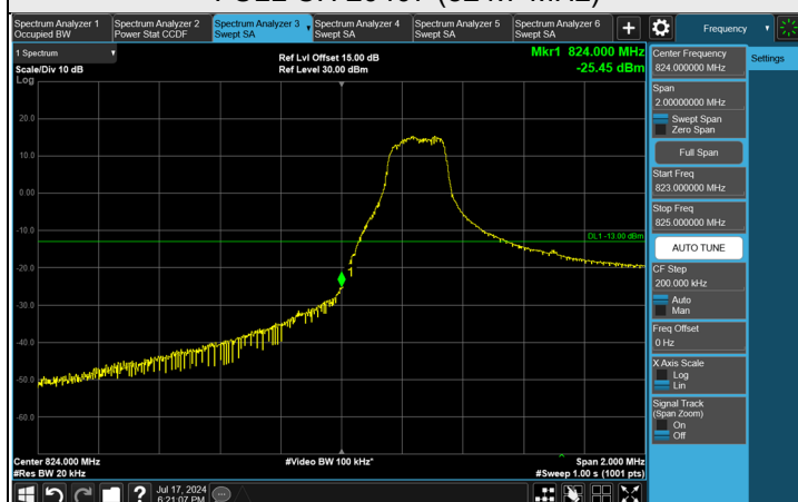
1RB CH 20407 (824.7 MHz)
