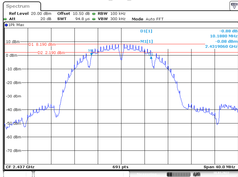
11B_Ant1_2437
