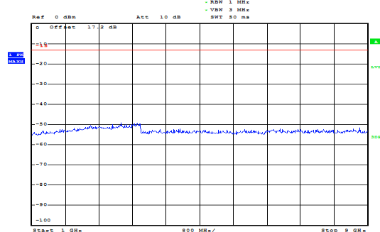
WCDMA Band V CH-Low 1GHz ~ 9GHz
