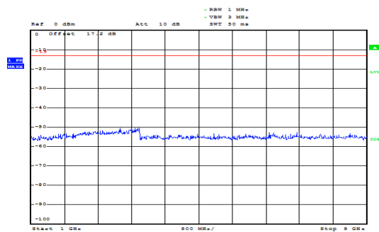
WCDMA Band V CH-Middle 1GHz ~ 9GHz
