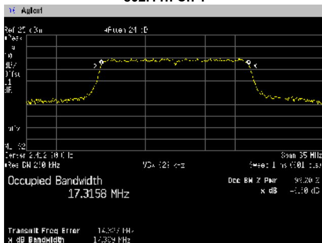
802.11n Ch 1
