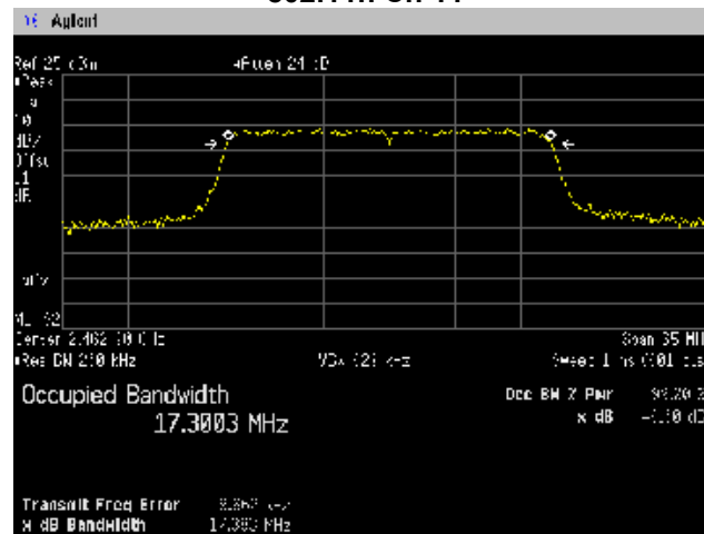
802.11n Ch 11
