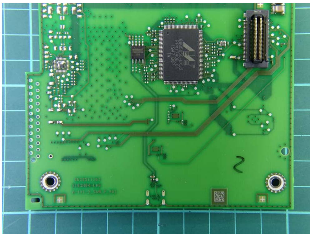
(48) EUT Photo
