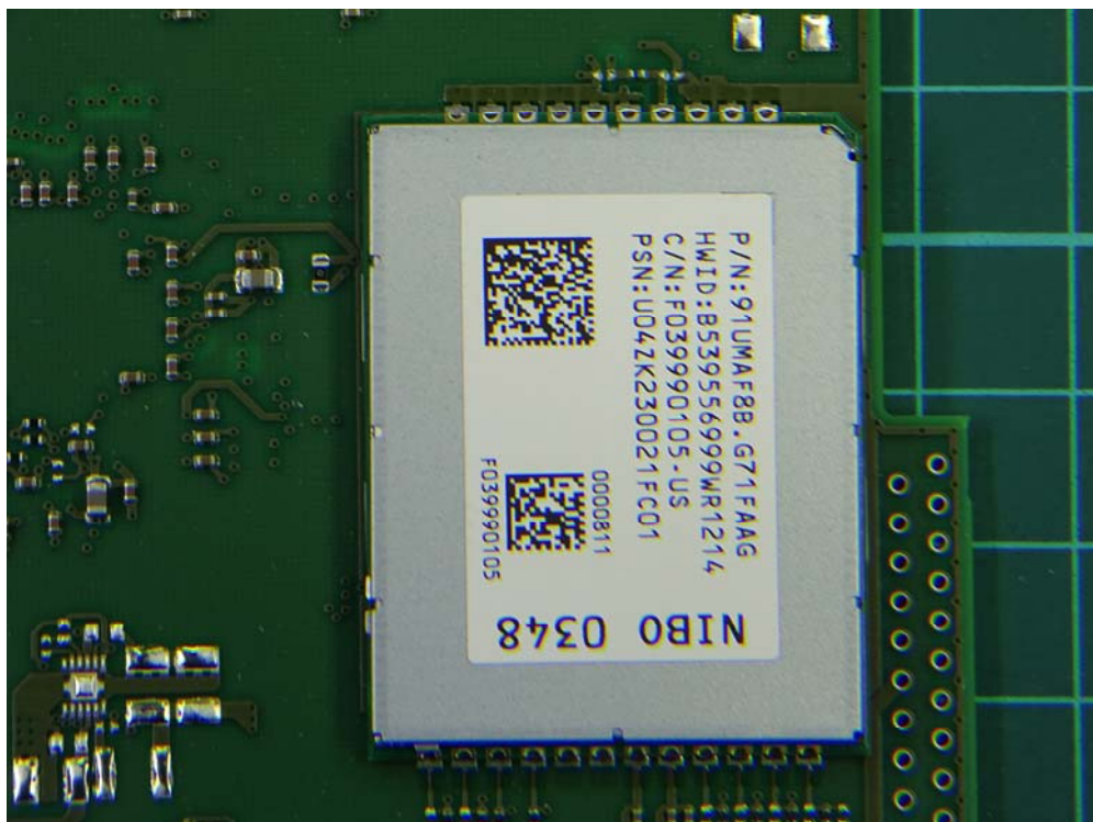
(52) EUT Photo
